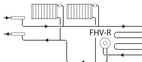
Fußbodentemperierung, Mischsystem: Heizkreis mit FHV-R am Ende der Fußbodenheizschlange.
