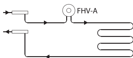
Fußbodenheizungssystem: Heizkreis mit FHV-A.
