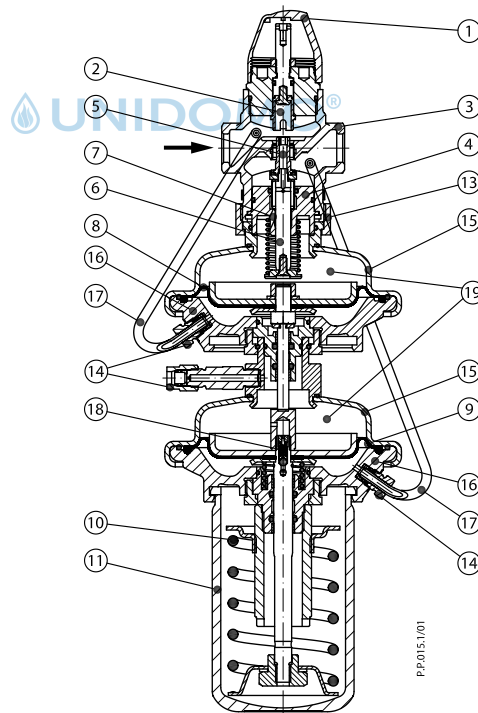
AVPQ 4 - Einbau im Rücklauf
