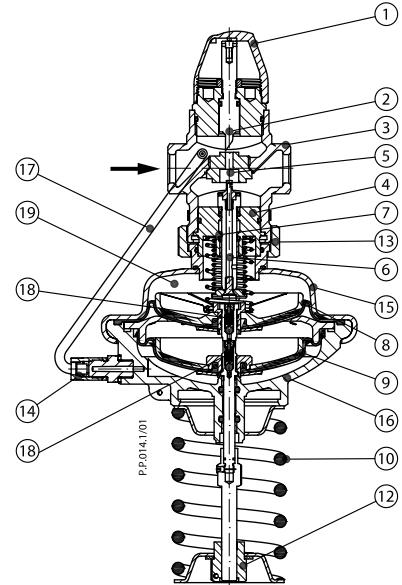
AVPQ (0,3-2,0 bar) - Einbau im Rücklauf
