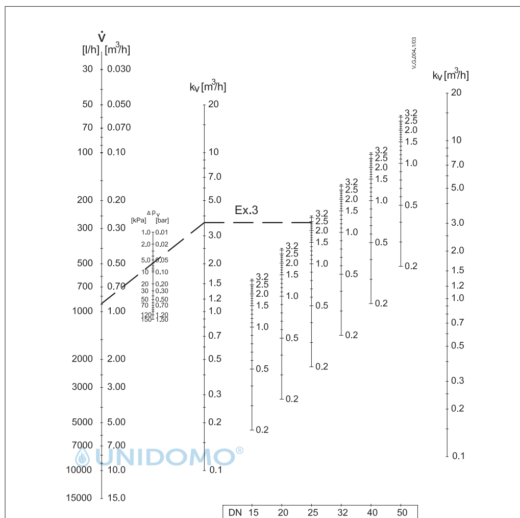
Abb. D: Dimensionierungsdiaqramm für das ASV-I, DN 15-50
