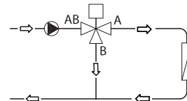
Abb. 4: Verteilventil
