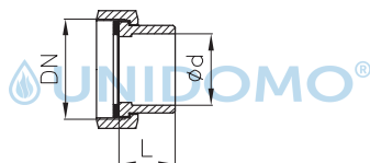
Anschweißenden
