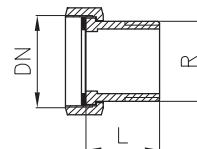
Anschraubenden
