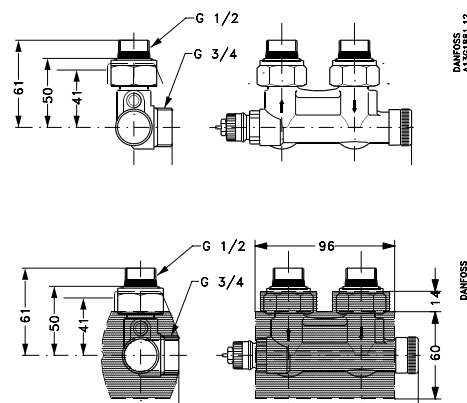
VHS Eckausführung, 1/2 und 3/4" Heizkörperanschluss
