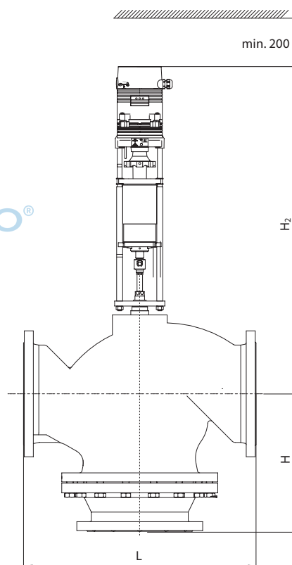
AMV(E) 855 + VF 3 (DN 200-300)
