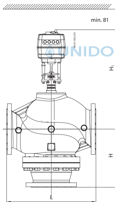
AMV(E) 685 + VF 3 (DN 200-300)
