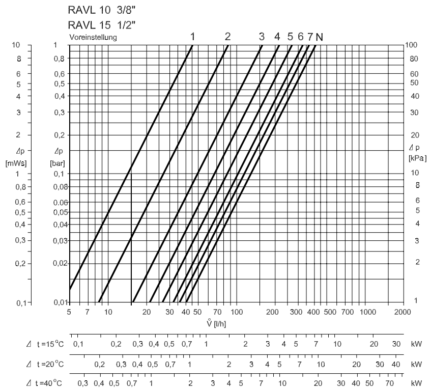
RAVL 15 Auslegungsdiagramm. Kapazitäten mit RA 2000 Fühlerelementen bei einem P-Band zwischen 0,5 K und 2 K.
