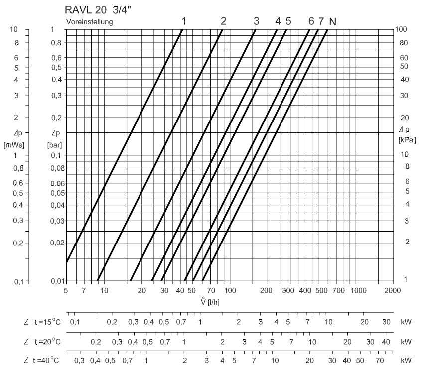
RAVL 20 Auslegungsdiagramm. Kapazitäten mit RA 2000 Fühlerelementen bei einem P-Band zwischen 0,5 K und 2 K.
