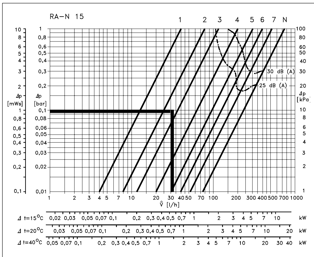
RA-N 15 Auslegungsdigramm. Kapazität mit RA 2000 Fühler bei einem P-Band zwischen 0,5 K und 2K.
