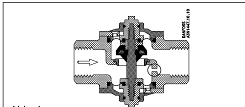
Abb. 4 Ventilkörper mit Bypass
