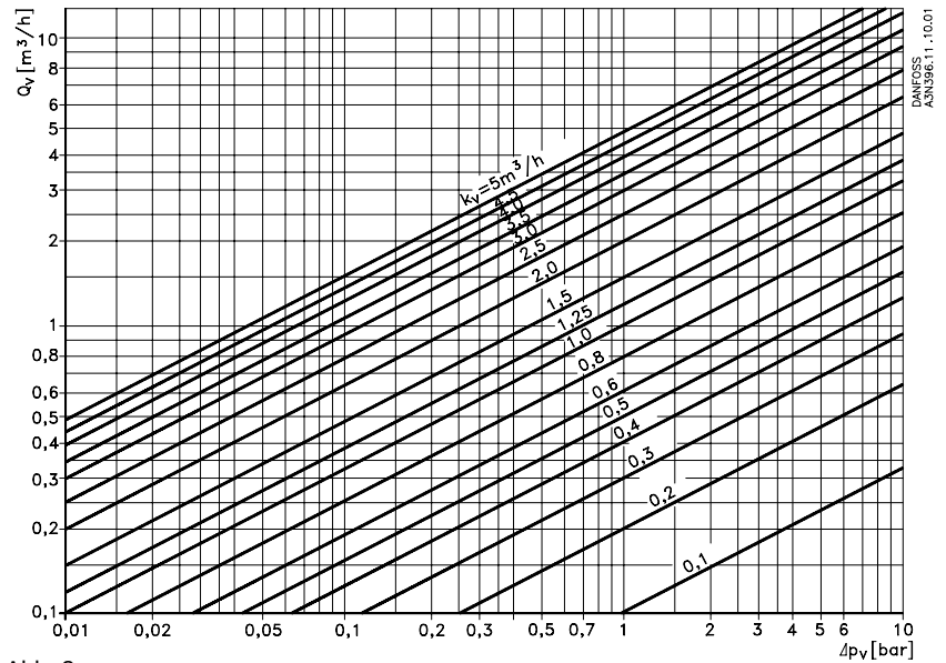
Abb. 2 Abhängigkeit von Wassermenge und Druckabfall über dem Ventil. Beispiel: Durchfluss 0,85 \text{ m}^3/\text{h} bei einem Druckabfall \Delta p von 1,5 bar. Für den k_v -Wert ergibt sich 0,7 \text{ m}^3/\text{h} .
