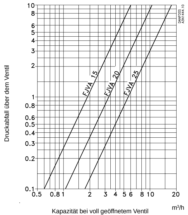
Abb. 4 Die Durchflussmenge der Ventile in völlig geöffnetem Zustand als Funktion des Druckabfalls \Delta p .
