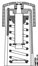
Abb. 1 Einstellungsteil mit Handrad, Einstellfeder und Einstellskala
