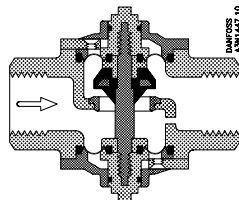
Abb. 2 Ventilkörper mit Düse, Ventilkegel, Dichtungselement und Bypassbohrung
