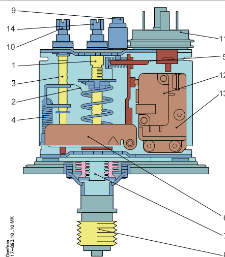
Prinzipzeichnung des BCP-Reglers
