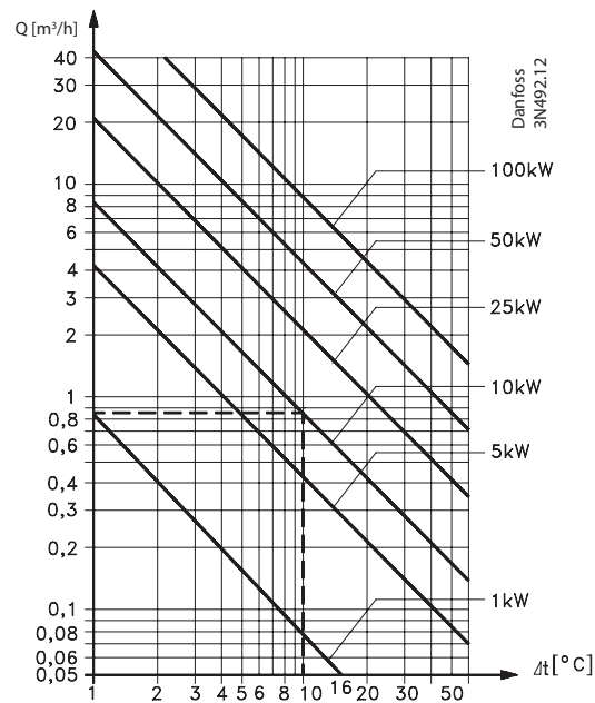
Fig.1 Erwärmung oder Abkühlung mit Wasser.
