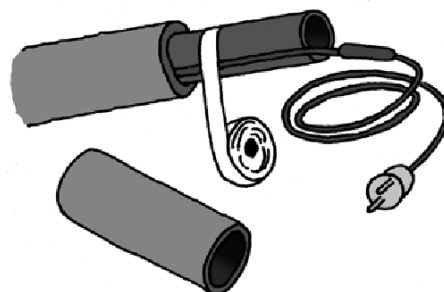
Montagebeispiele
