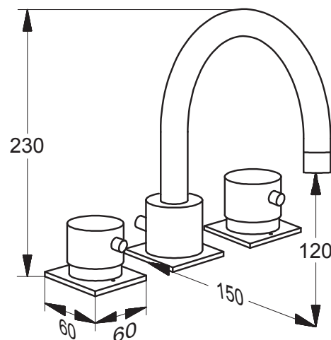
3Loch-Waschtischbatterie mit Ab- und Überlauf verchromt F1261AA
