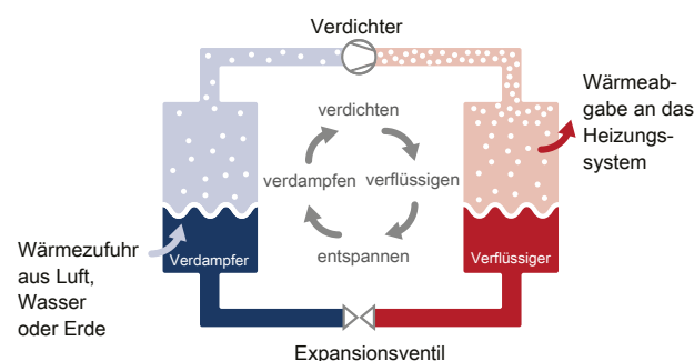
Abb. 1: Kältekreislauf
