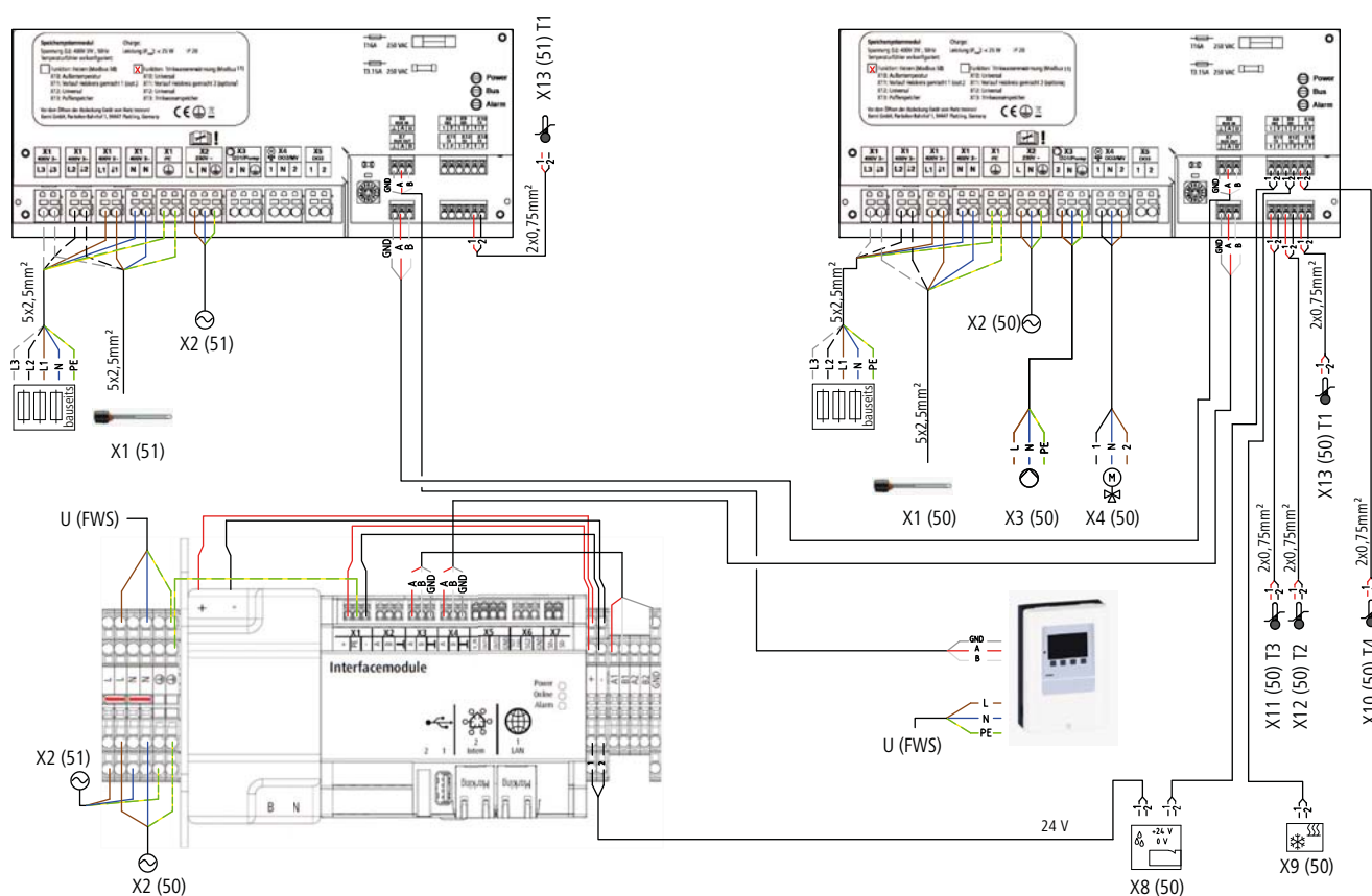
Abb. 30: Elektroinstallation Inneneinheit
