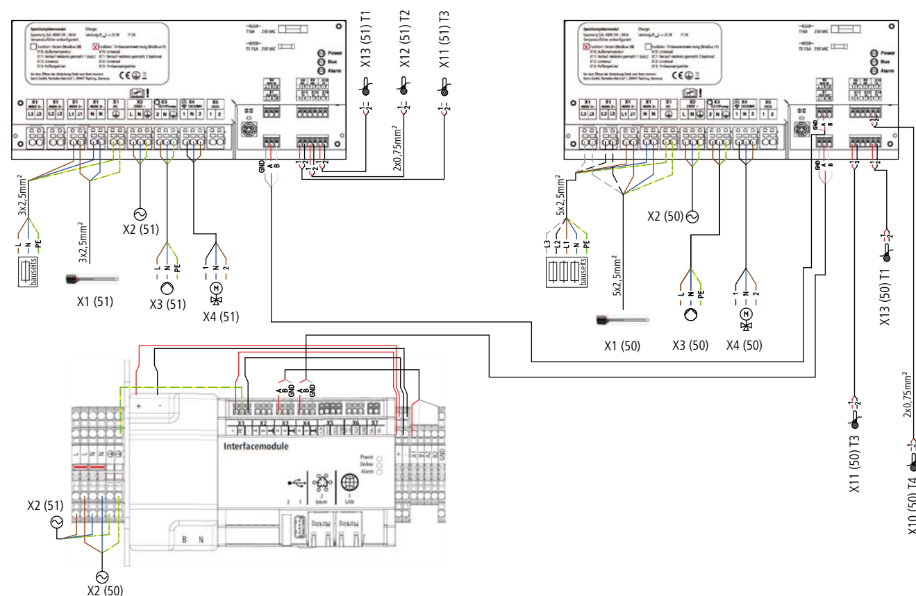
Abb. 24: Elektroinstallation Inneneinheit
