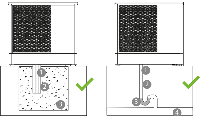
Abb. 7: Kondensatablauf: Versickerung oder Entwässerungsrohr
