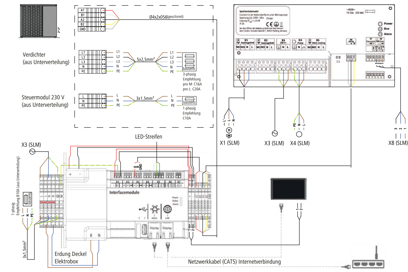
Abb. 24: Elektroinstallation Inneneinheit
