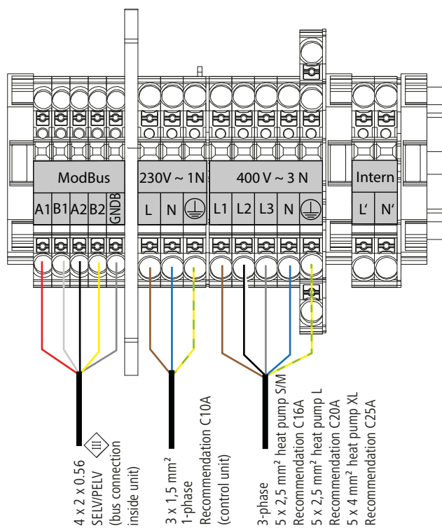
Abb. 13: Anschlussklemmen
