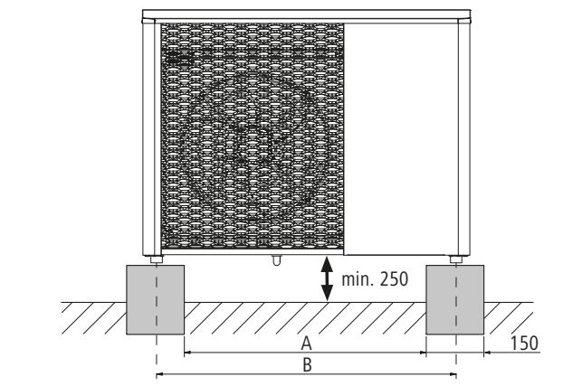
Abb. 8: Montage: Betonfundament
