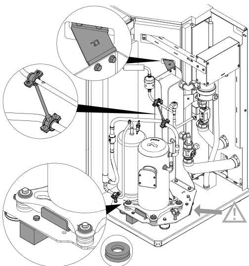
Abb. 15: Transportsicherungen entfernen
