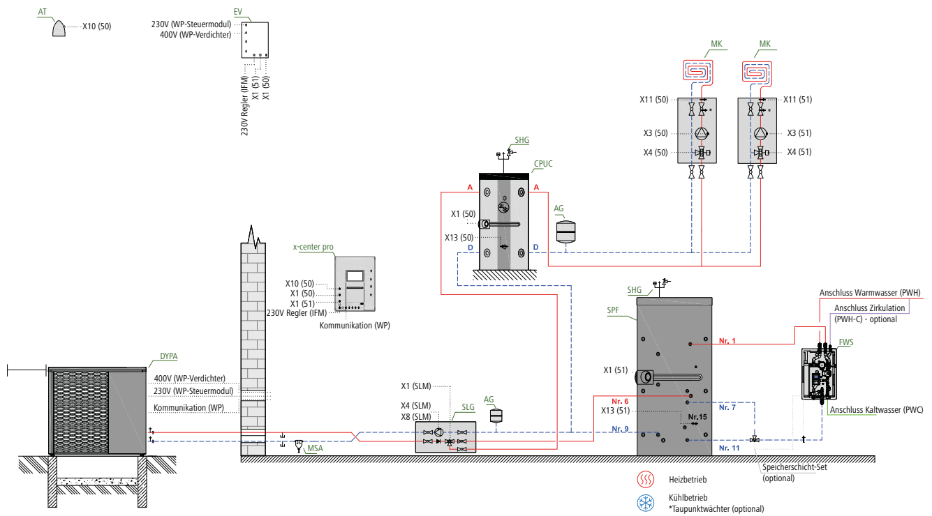
Abb. 25: Hydraulikschemata
