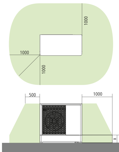
Abb. 4: Schutzbereich: Aufstellung vor einem Gebäude
