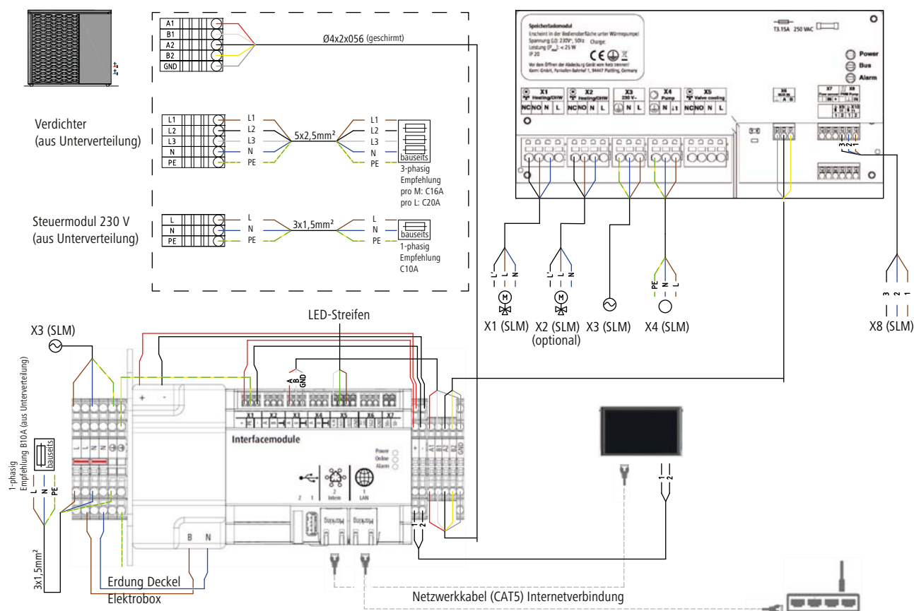
Abb. 27: Elektroinstallation Inneneinheit
