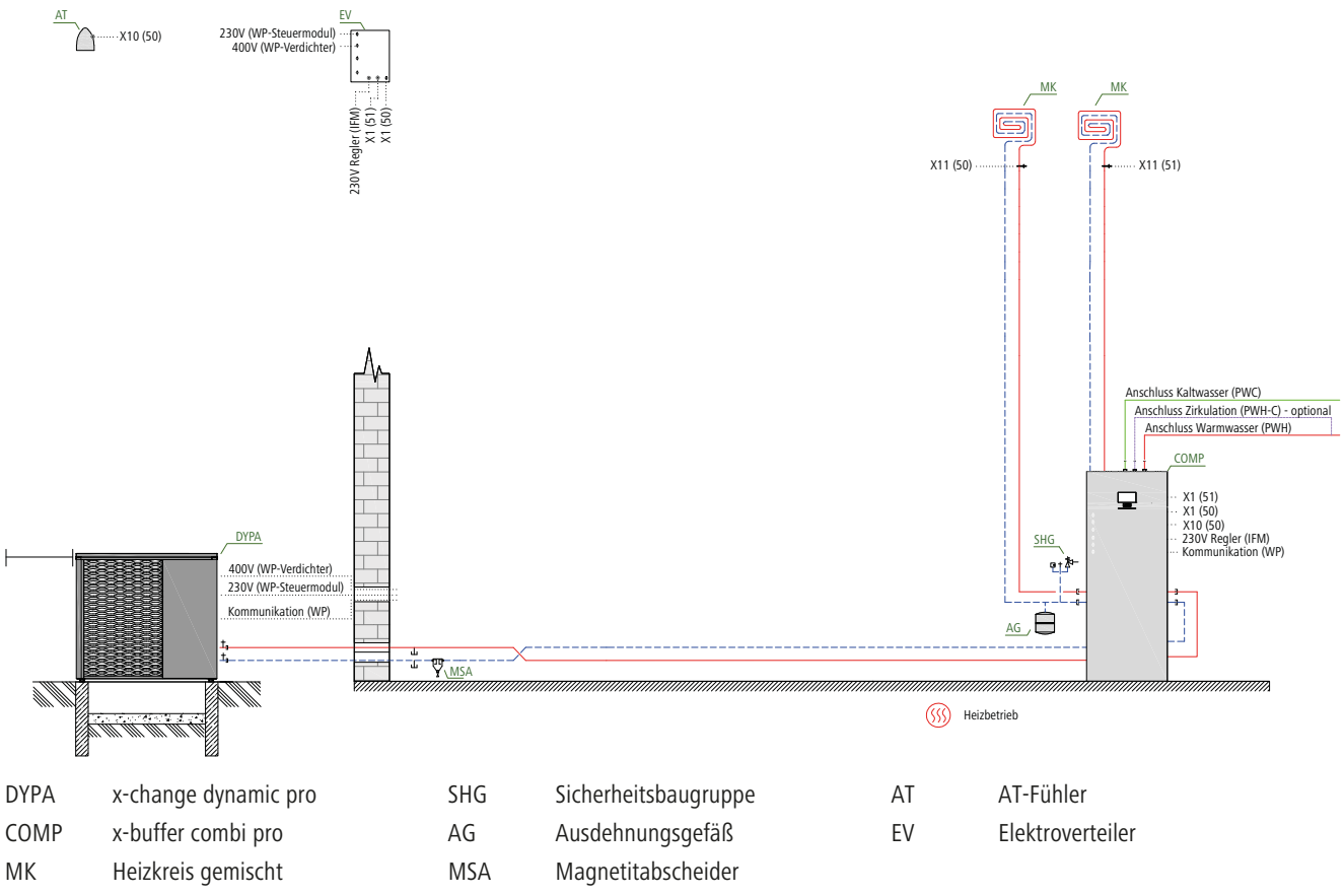
Abb. 22: Hydraulikschem
