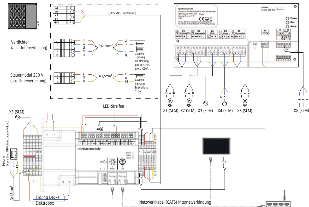
Abb. 30: Elektroinstallation Inneneinheit
