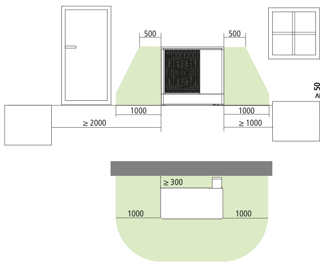
Abb. 4: Schutzbereich: Aufstellung vor einem Gebäude
