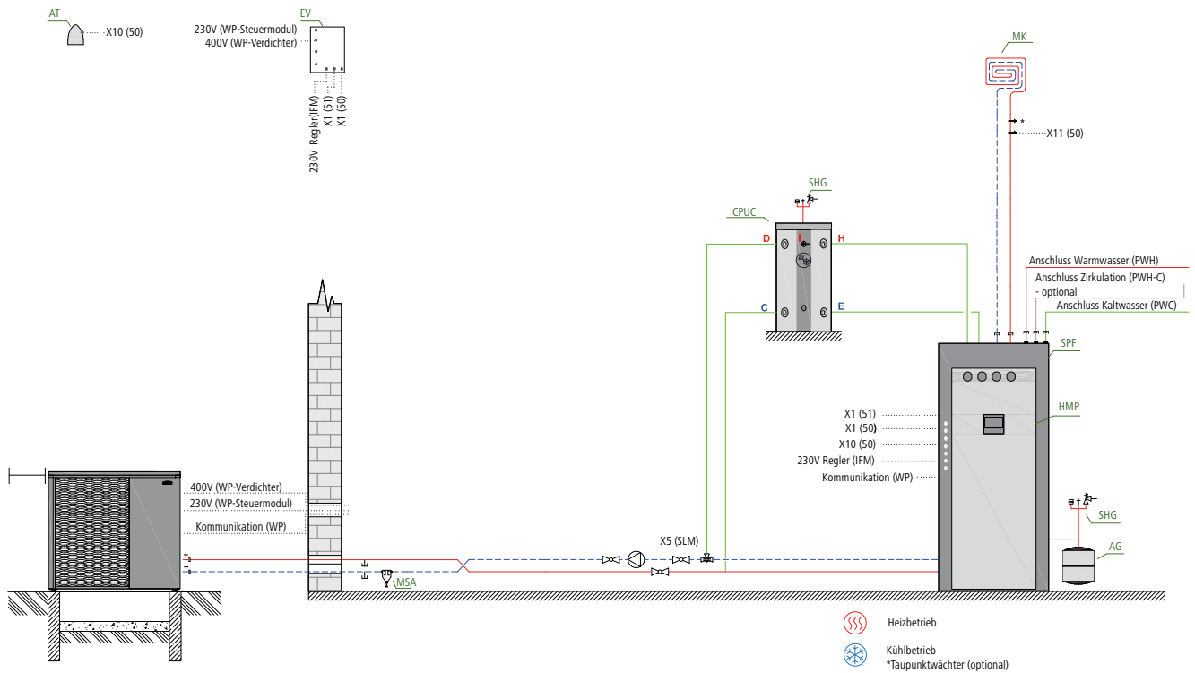
Abb. 28: Hydraulikschema
