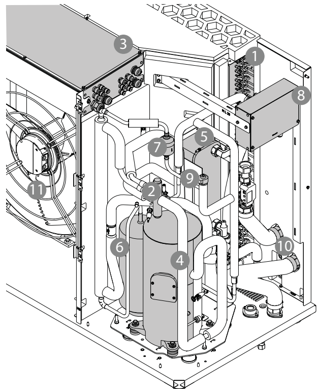
Abb. 2: Komponentenübersicht
