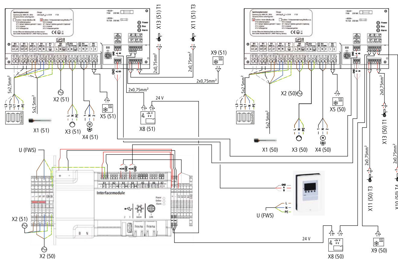
Abb. 27: Elektroinstallation Inneneinheit
