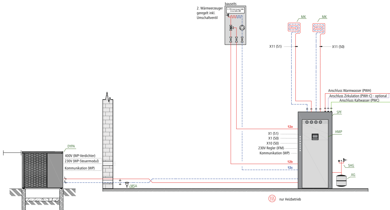
Abb. 32: Hydraulikschema
