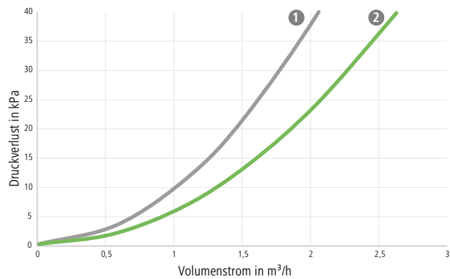
Abb. 21: Druckverlust der Sekundärseite der Wärmepumpe
