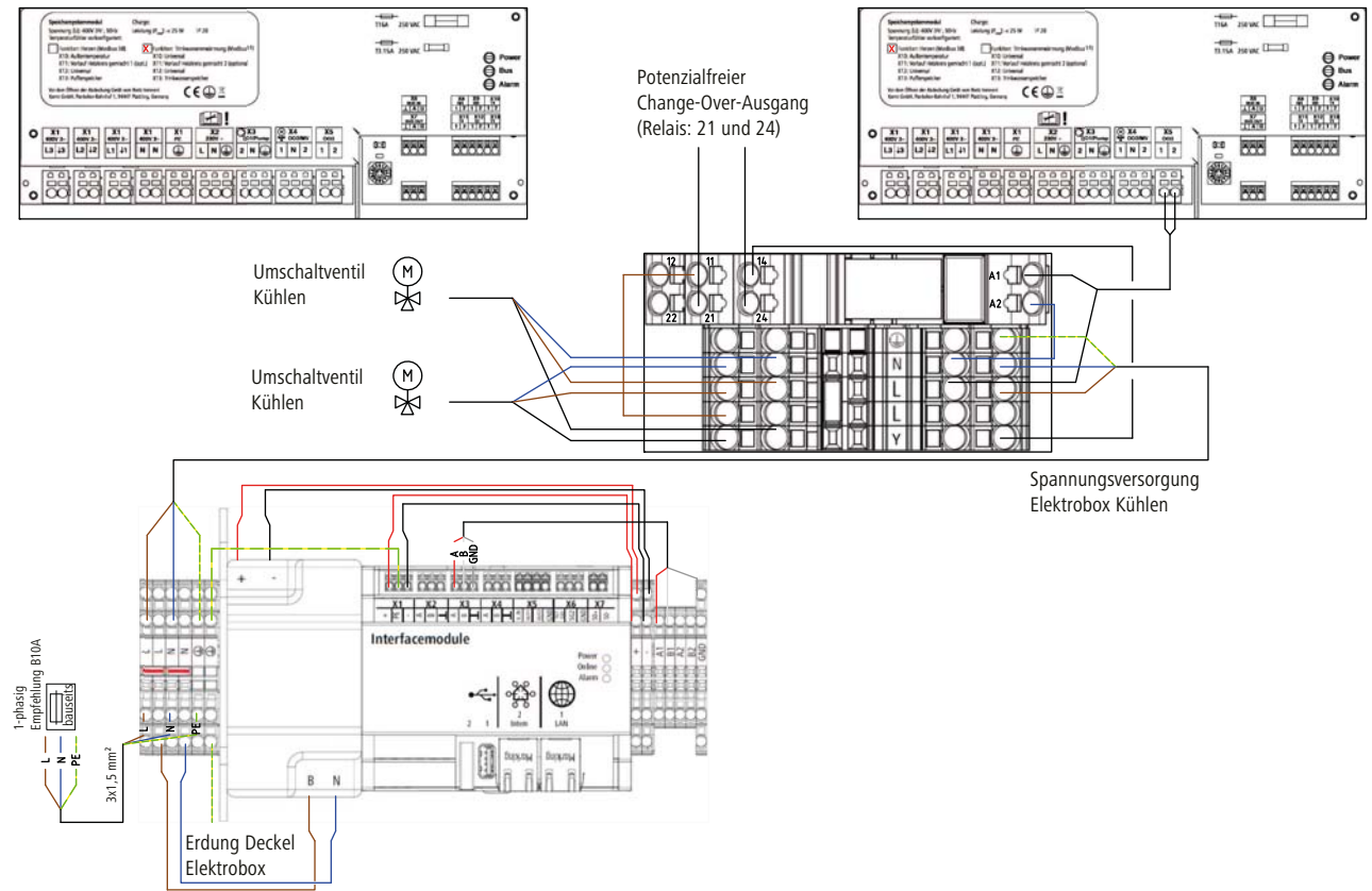
Abb. 31: Elektroinstallation Inneneinheit
