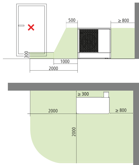
Abb. 5: Schutzbereich: Eckaufstellung [mm]
