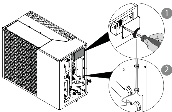
Abb. 12: Öffnen der Anschlussbox - Einführung und Anschluss der Leitungen
