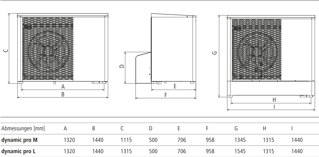
Abb. 16: Abmessungen der Wärmepumpe
