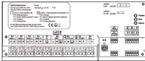
Abb. 35: Elektroinstallatin Inneneinheit
