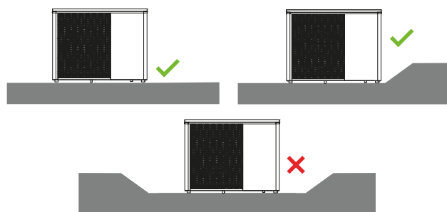
Abb. 6: Aufstellung in Senken
