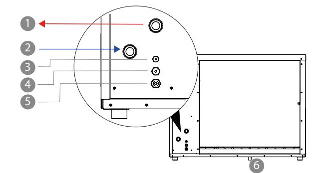
Abb. 9: Anschlüsse auf der Rückseite
