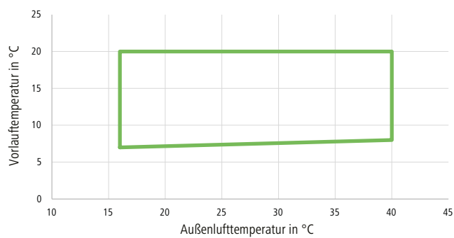
Abb. 20: Kühlbetrieb
