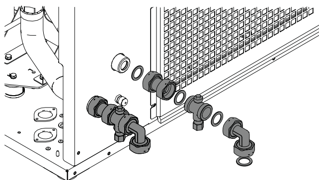
Abb. 10: Montage Frostschutzventil
