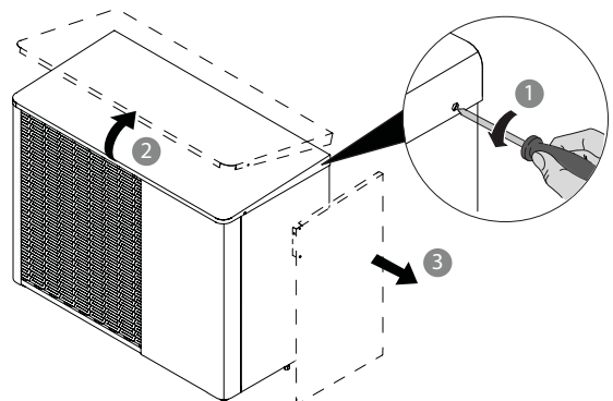
Abb. 11: Entfernen der oberen und seitlichen Abdeckung
