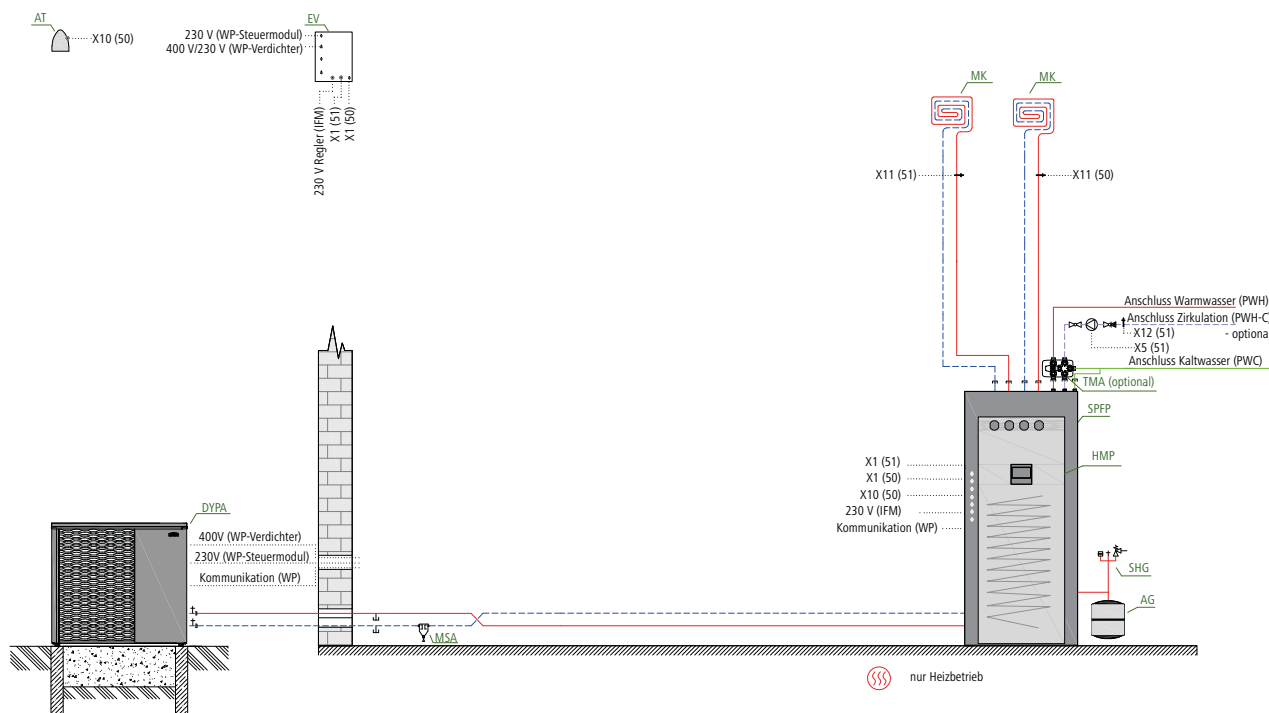
Abb. 13: Hydraulikschema
