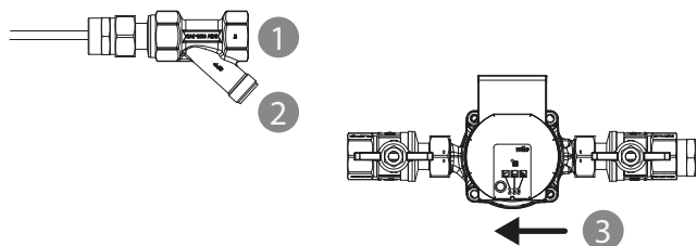
Abb. 9: Zirkulationsset
