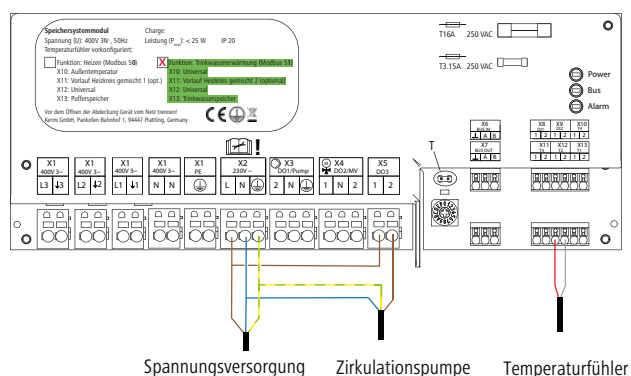
Abb. 14: Anschlussbild
