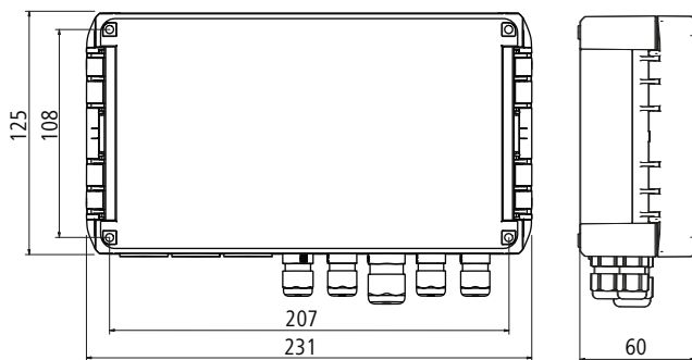
Abb. 4: Abmessungen und Bohrmaße
