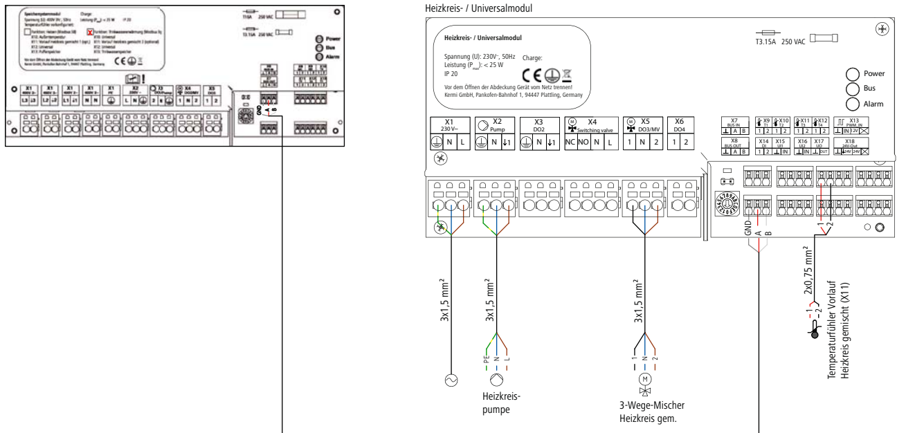
Abb. 14: Elektroinstallation Heizkreis-/Universalmodul
