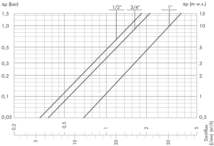
Empfohlene Durchflussmengen für einen stabilen Betrieb und eine Präzision von ±2°C
