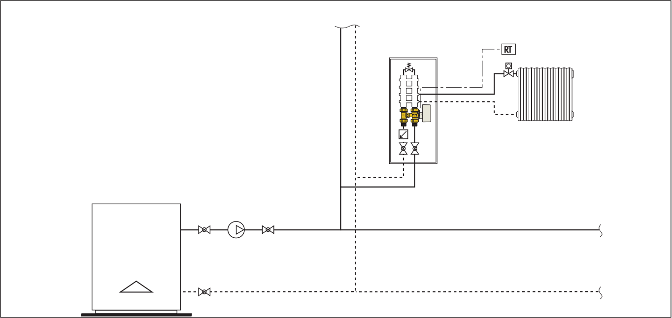
System mit Dreiwege-Zonenventilen mit Bypass-T-Stück und AUTOFLOW®, Serie 6444
