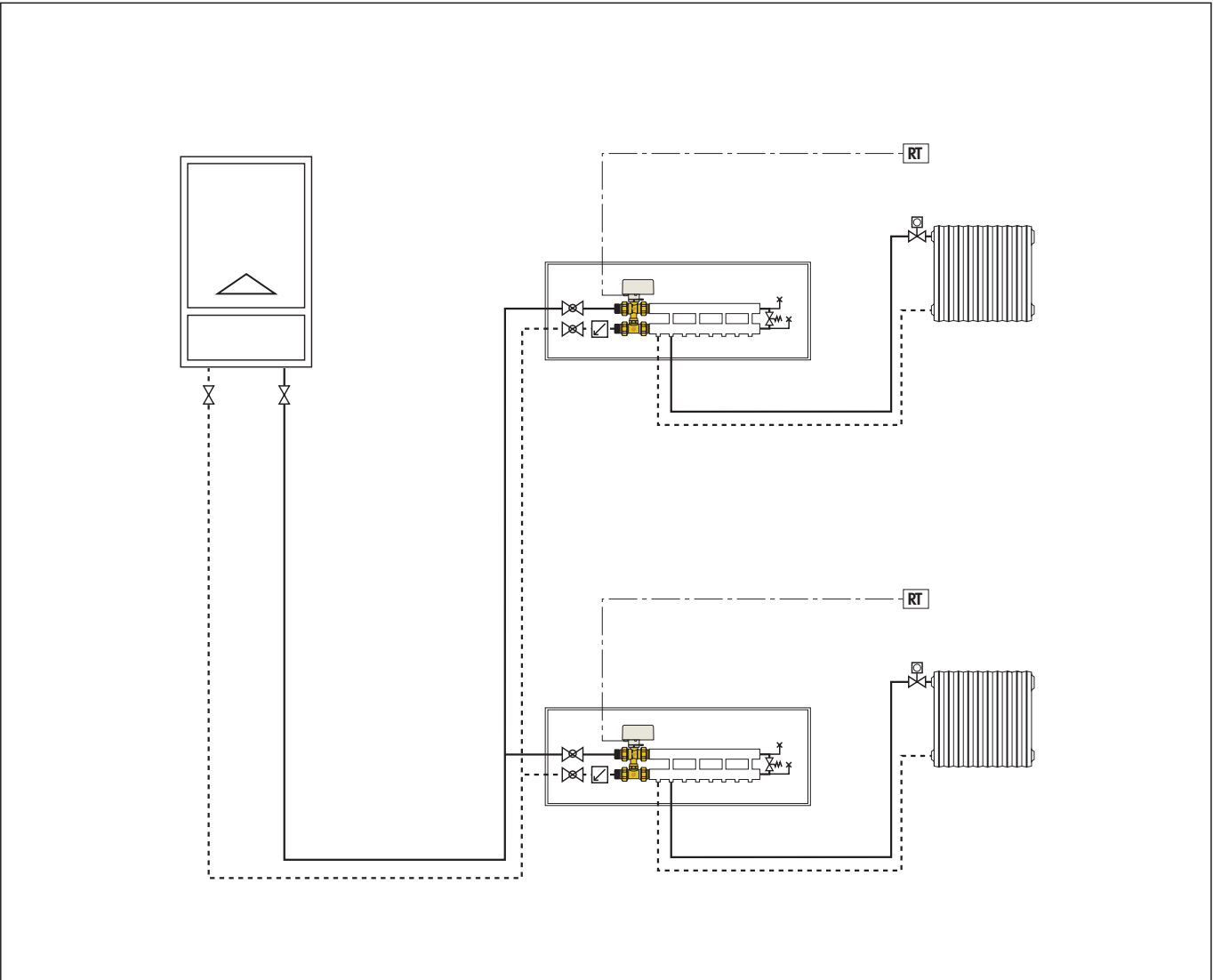
Unabhängige Anlage mit Dreiwege-Zonenventilen mit Bypass-T-Stück und AUTOFLOW®, Serie 6444
