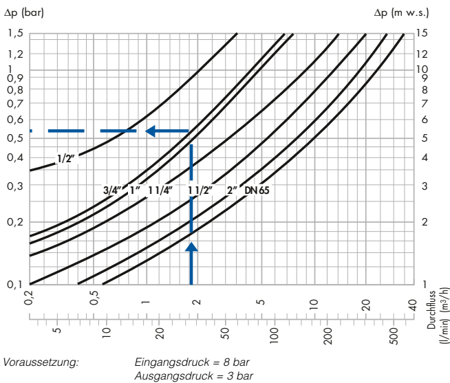
Diagramm 2 (Druckverlust)
