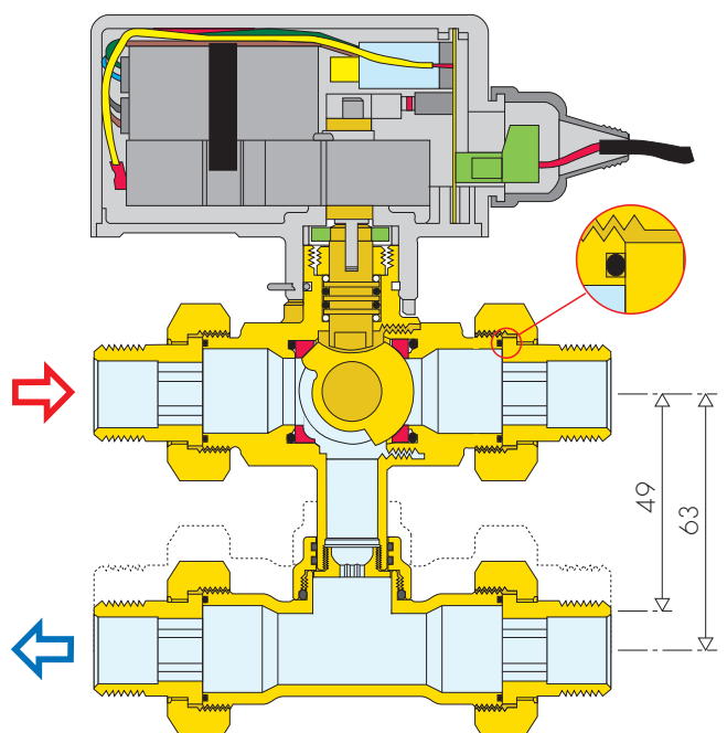
3-Wege-Ventil mit Bypass Art.Nr. 648950
