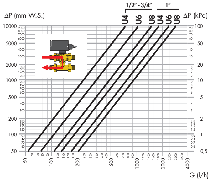
3-Wege-Zonenventil Serie 6480 in Funktionsweise "BY-PASS" mit Bypass-T-Stück Serie 6490 einschließlich bei der Bestellung anzugebender U4 - U6 - U8
