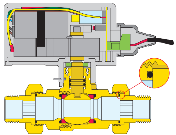
2-Wege-Ventil Serie 6470
