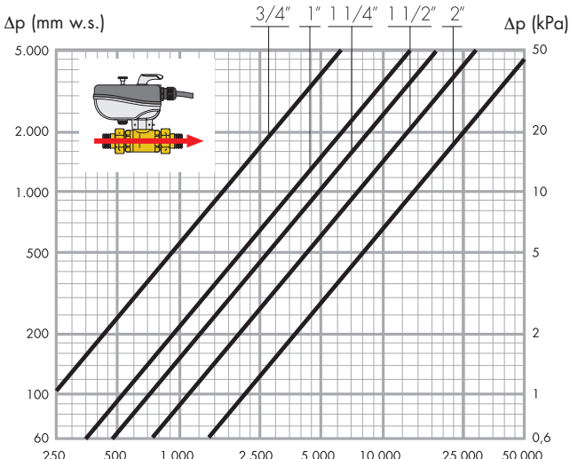
Zweiwegeventil Serie 638
