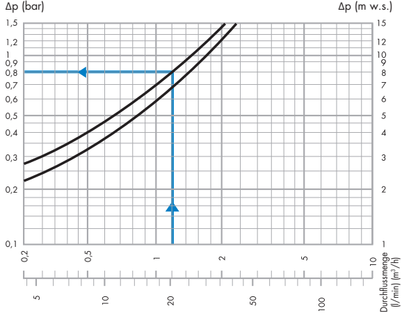
Diagramm 2 (Druckabfall)
