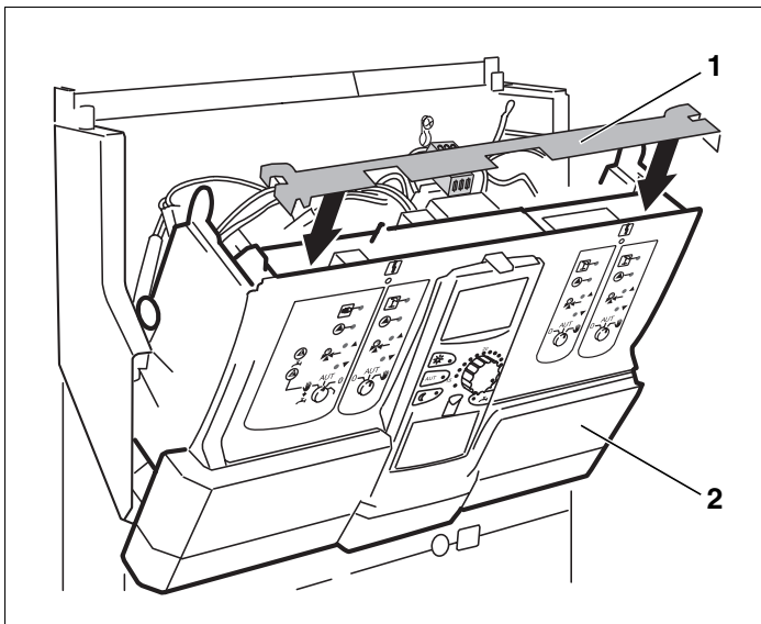
Bild 9 Querleiste einsetzen
