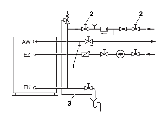
Abb. 11 Installation nach DIN 1988 (Prinzipabbildung)
