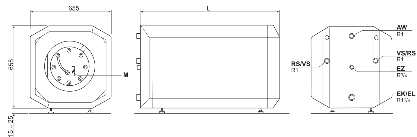
Abb. 2 Abmessungen und Anschlüsse (Maße in mm)
