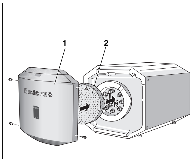
Abb. 17 Wärmeschutz und Vorderwand montieren
