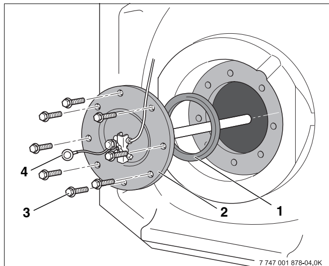
Abb. 16 Handlochdeckel einsetzen
