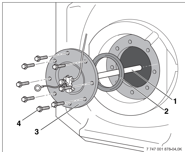
Abb. 13 Handlochdeckel demontieren
