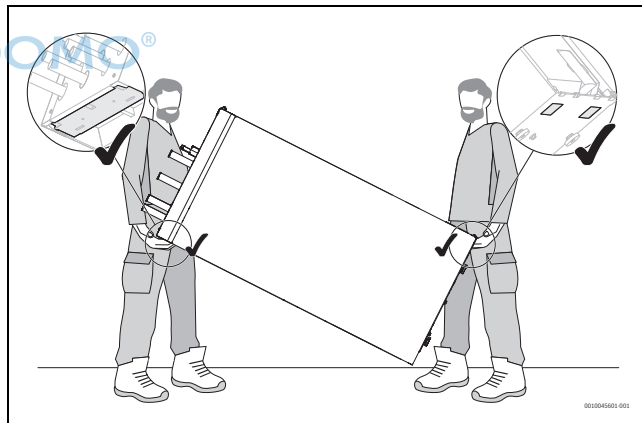
Bild 10 Inneneinheit anheben
