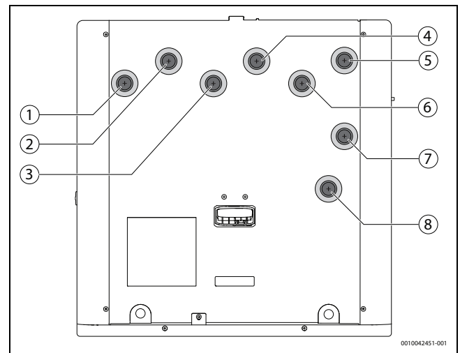
Bild 16 Hydraulische Anschlüsse
