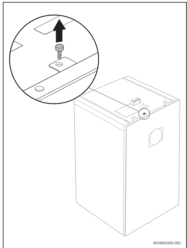
Bild 11 Sicherungsschraube lösen
