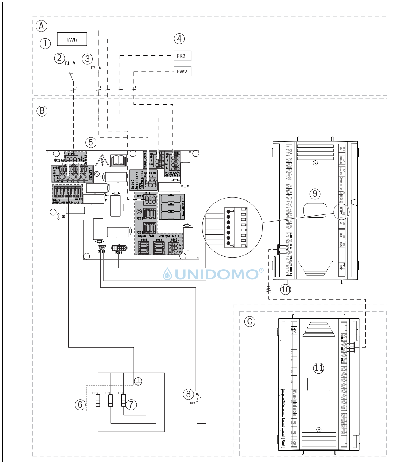
Bild 53 Spannungsversorgung Inneneinheit
