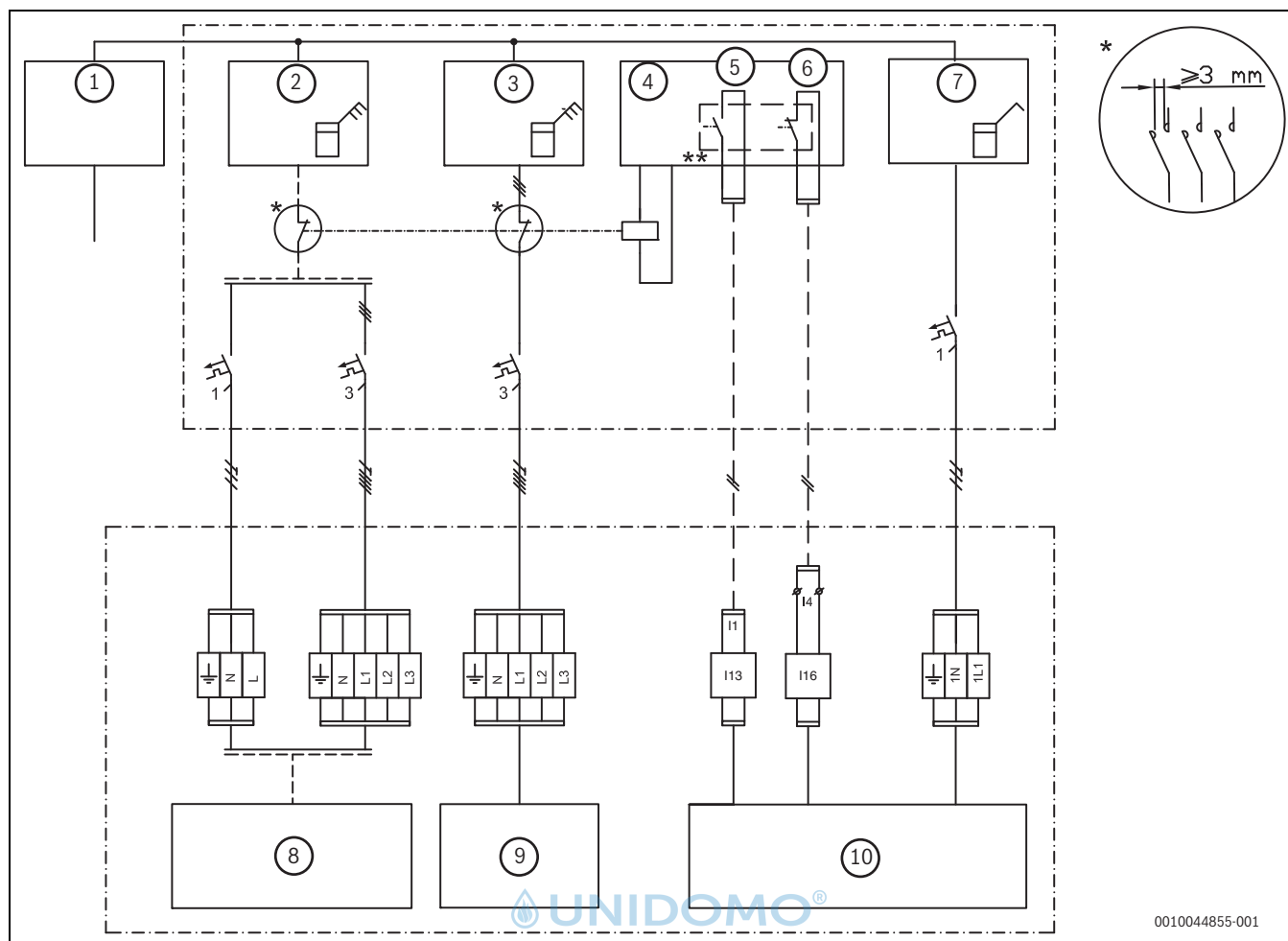
Bild 45 Alternative Lösung
