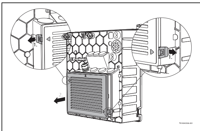
Bild 30 Abdeckung abnehmen
