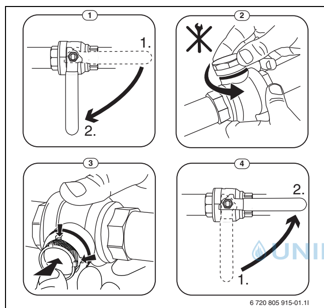
Bild 50 Filterventil reinigen
