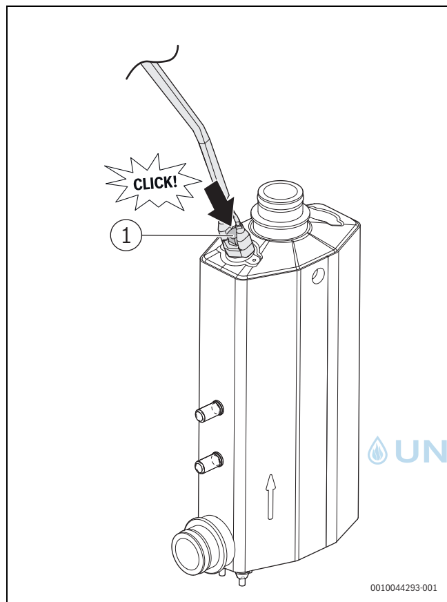
Bild 47 Elektrischer Zuheizer
