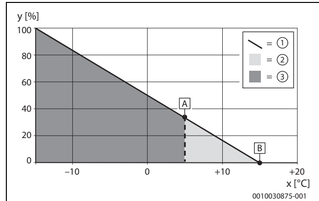
Bild 2 Außentemperatur alternativ
