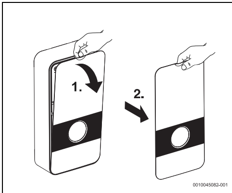
Bild 10 Frontblende abnehmen
