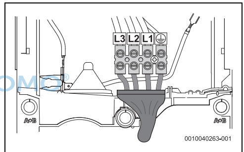
Bild 39 Anschluss unten für kurze Kabel
