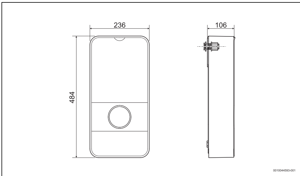
Bild 2 Abmessungen in mm
