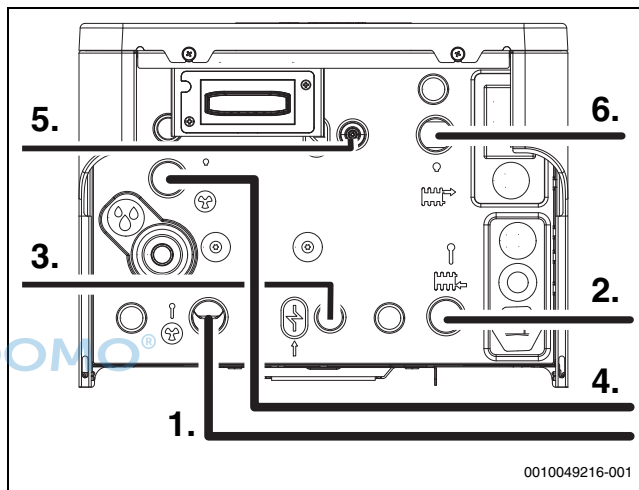
Bild 14 Rohranschlüsse
