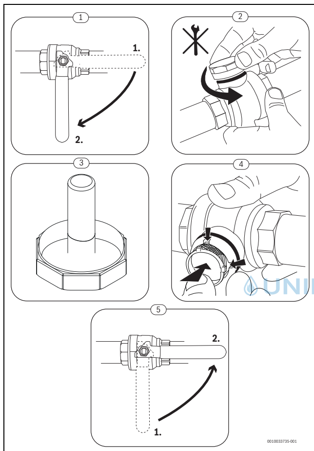
Bild 40 Siebreinigung
