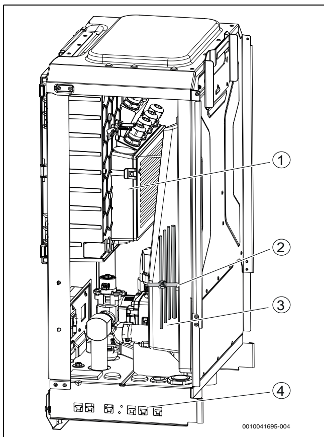
Bild 26 Kabelführung
