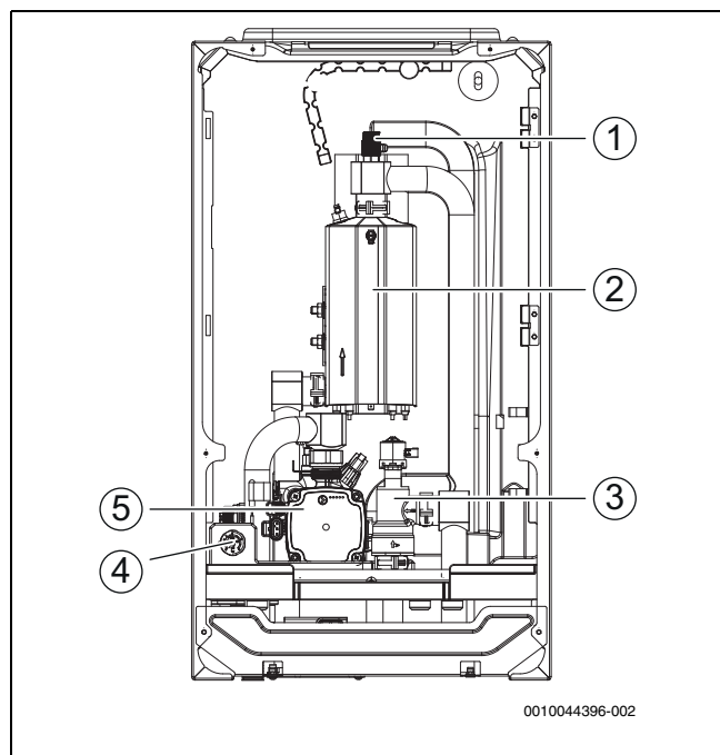
Bild 5 Komponenten
