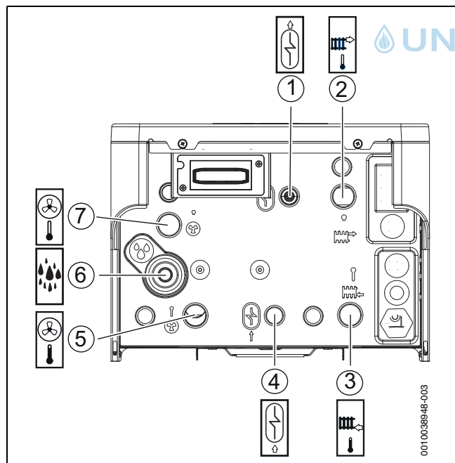
Bild 6 Rohranschlüsse
