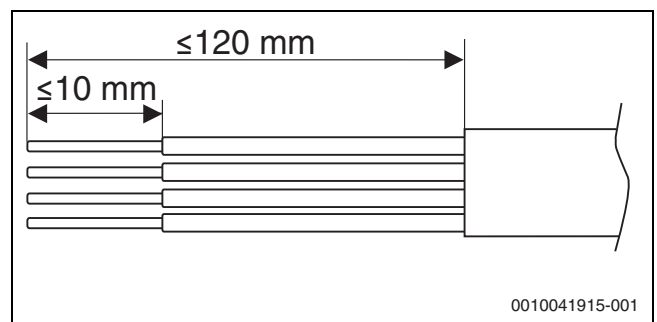
Bild 27 Abisolierung CAN-BUS
