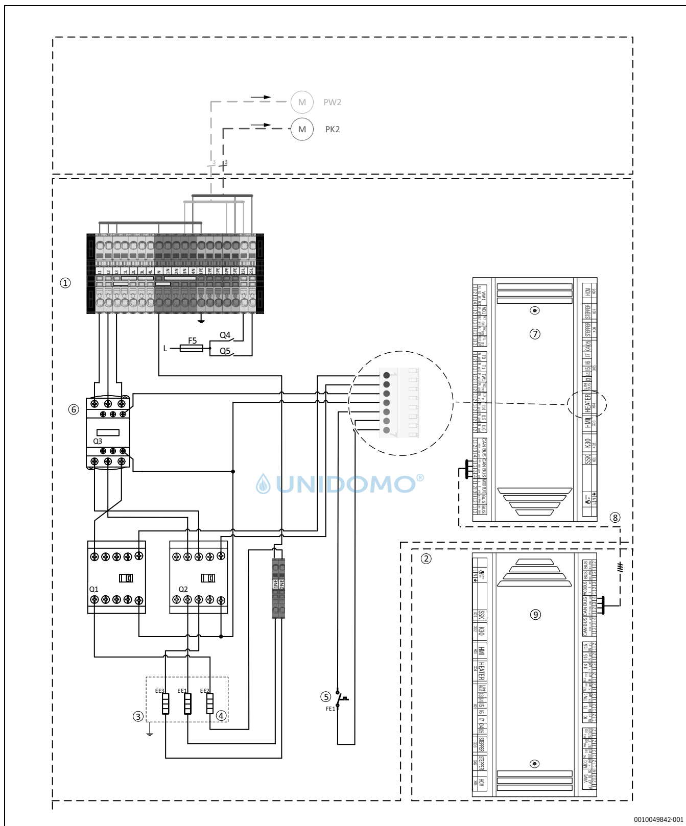
Bild 52 Spannungsversorgung Inneneinheit
