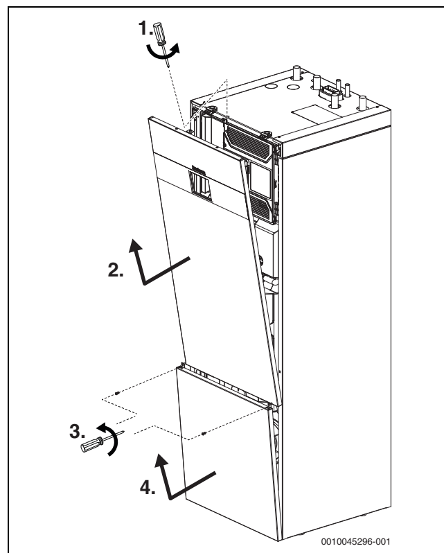
Bild 16 Demontage der Frontseite
