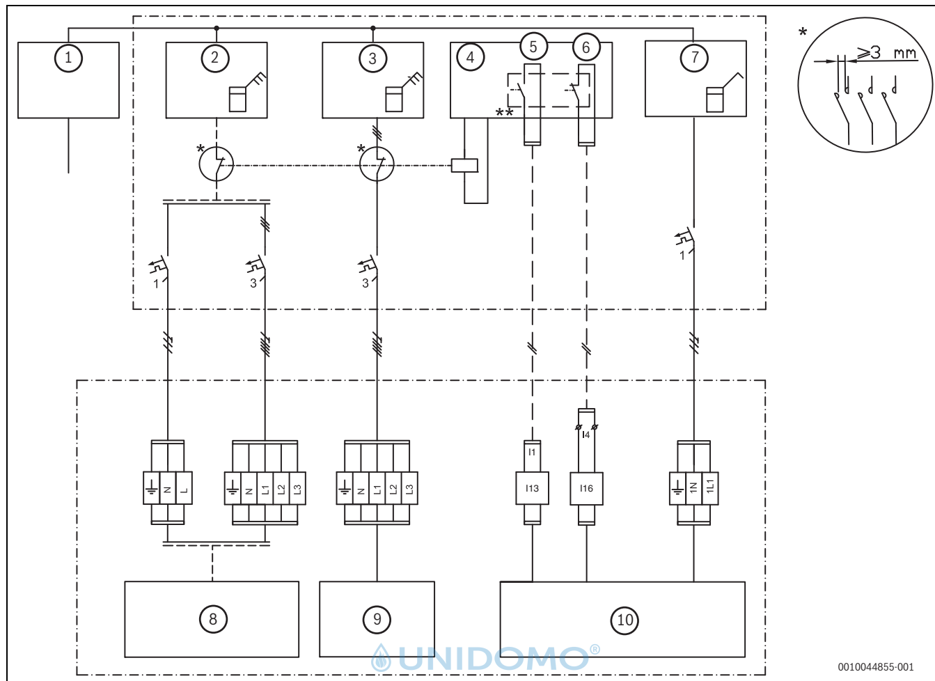
Bild 41 Alternative Lösung
