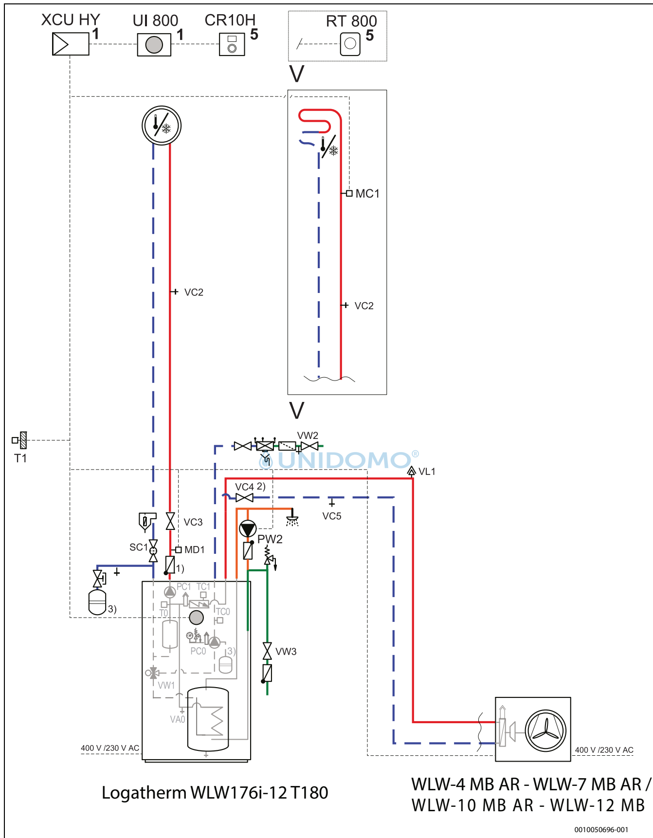
Bild 46 Tower Inneneinheit, Wärmepumpe (ODU), ein ungemischter Heizkreis
