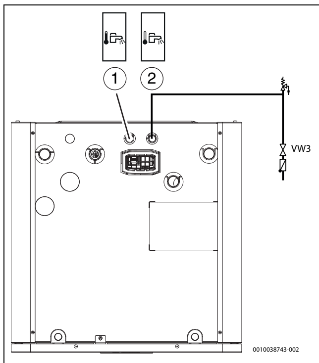
Bild 23 Warmepumpenanschlüsse Trinkwasser
