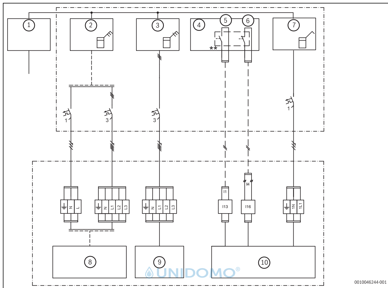
Bild 40 Empfohlene Lösung
