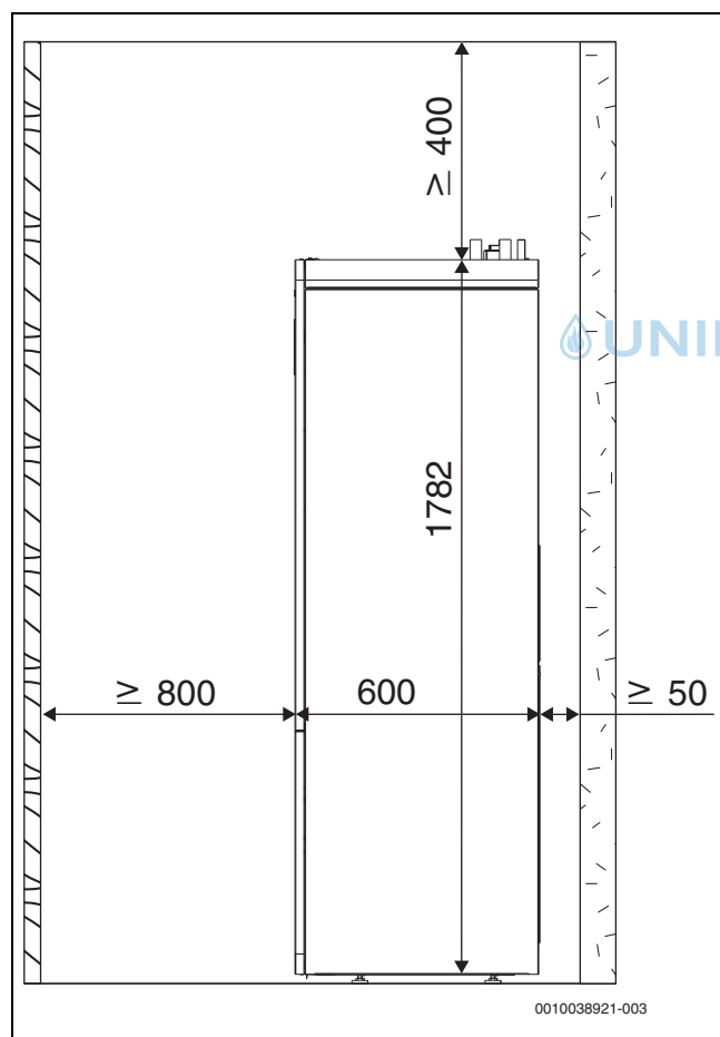
Bild 2 Mindestabstand (mm)
