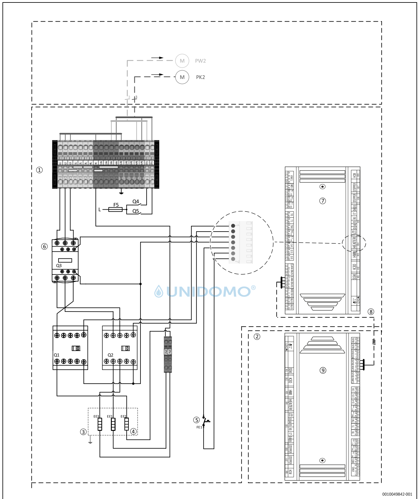
Bild 50 Spannungsversorgung Inneneinheit
