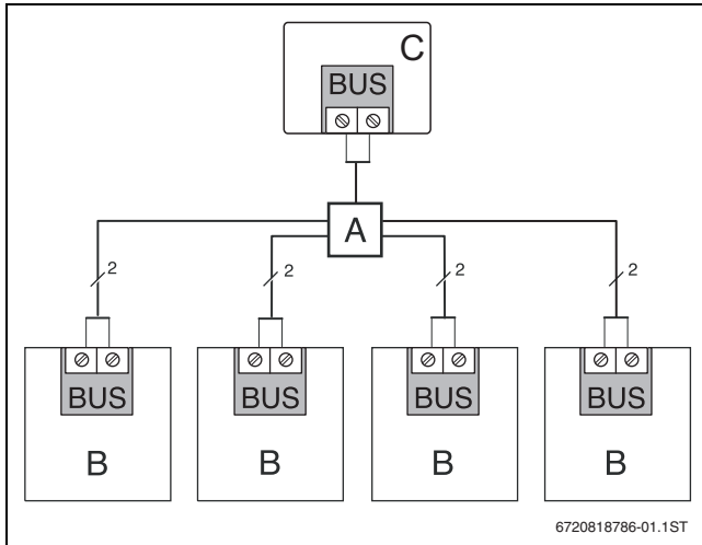
Bild 54 BUS-Leitungen anschließen
