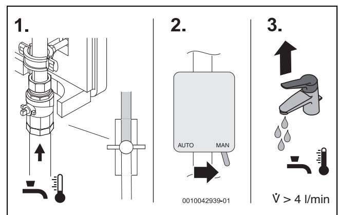
Bild 57 Vorbereitungen
