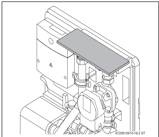
Bild 17 Anschlüsse oben während der Montagearbeiten abdecken
