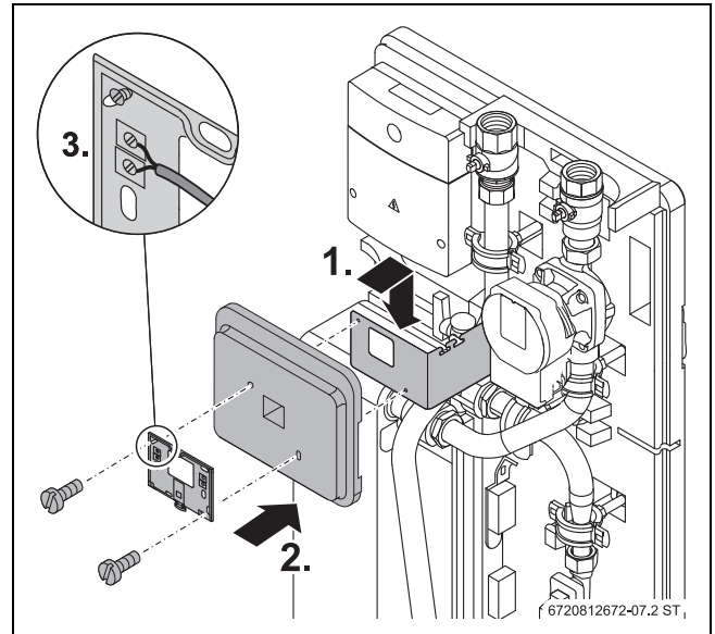
Bild 38 Distanzstück und Sockel der Bedieneinheit montieren
