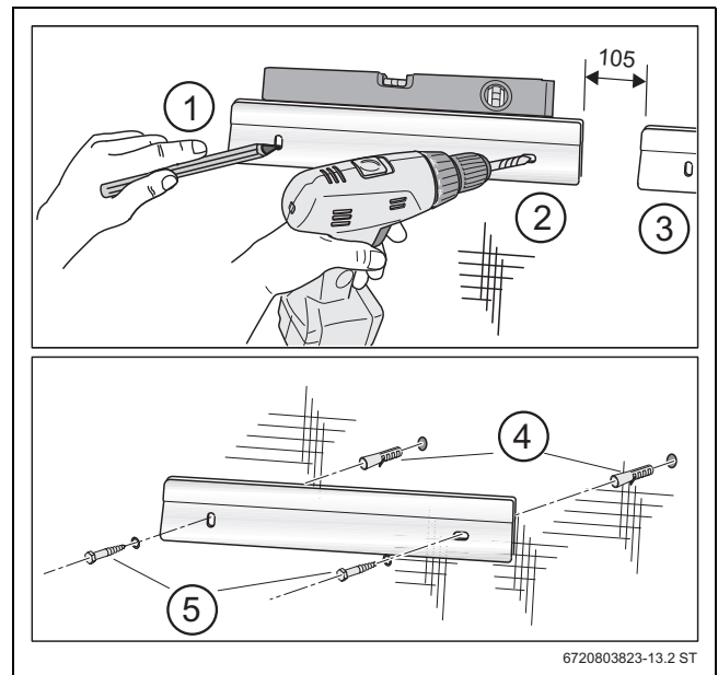
Bild 18 Wandhalter montieren (Maß in mm)
