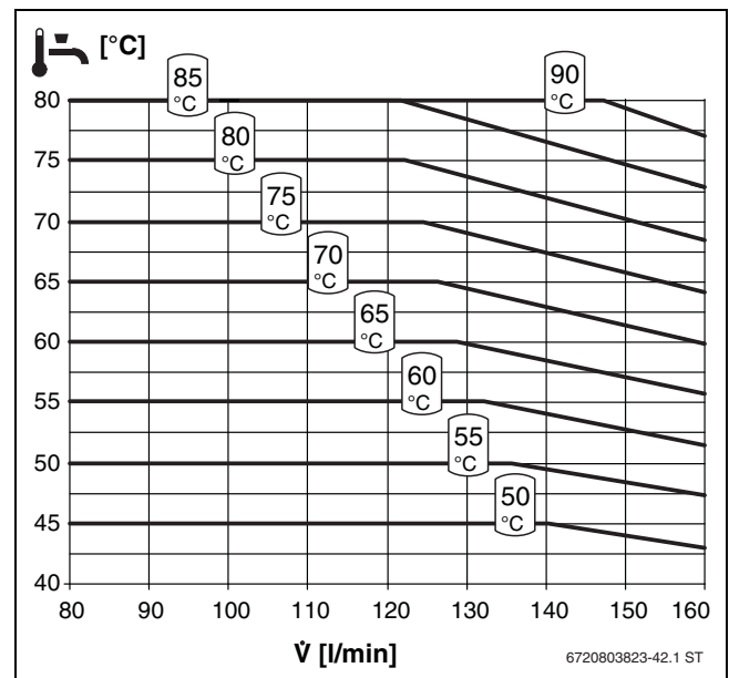
Bild 64 Temperaturverhalten Kaskade FS160S/3E
