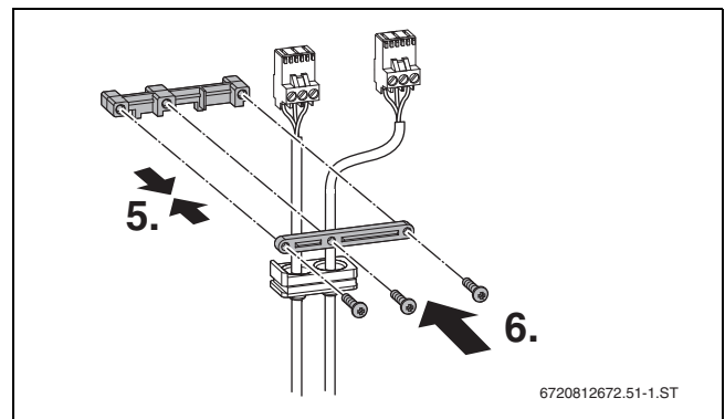
Bild 52 Zugenlastung montieren
