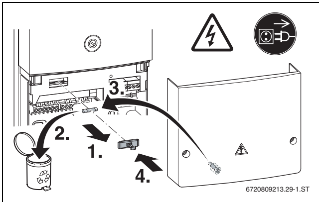
Bild 68 Sicherung tauschen
