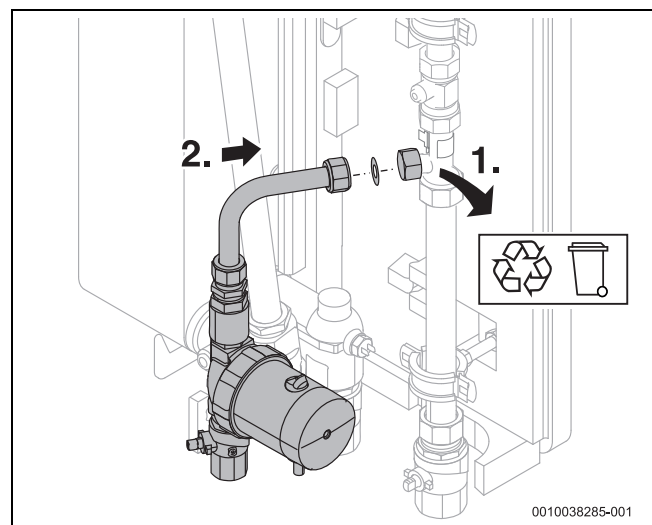
Bild 22 Zirkulationsstrang montieren
