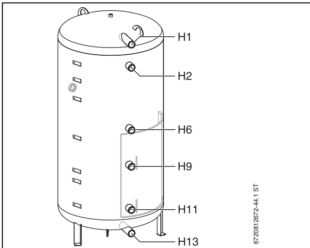
Bild 36 Pufferspeicher als Solarspeicher (getrenntes Volumen), Hydraulik (→Bild 6, Seite 6)
