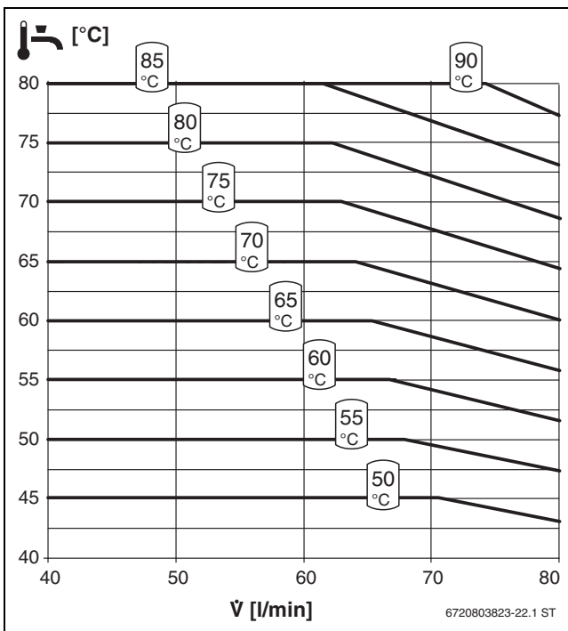
Bild 62 Temperaturverhalten Kaskade FS80/3E
