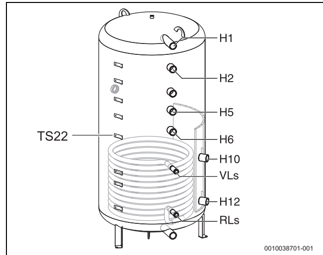
Bild 34 Pufferspeicher mit Bereitschafts- und Solarvolumen (gemeinsames Volumen), Hydraulik (→ Bild 4, Seite 5)
