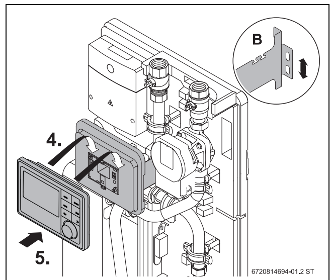
Bild 39 Bedieneinheit montieren
