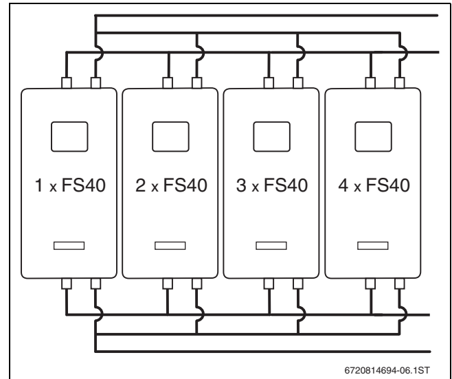
Bild 32 Stationen bauseits verbinden (Beispiel: Anschlussseite rechts mit FS40)
