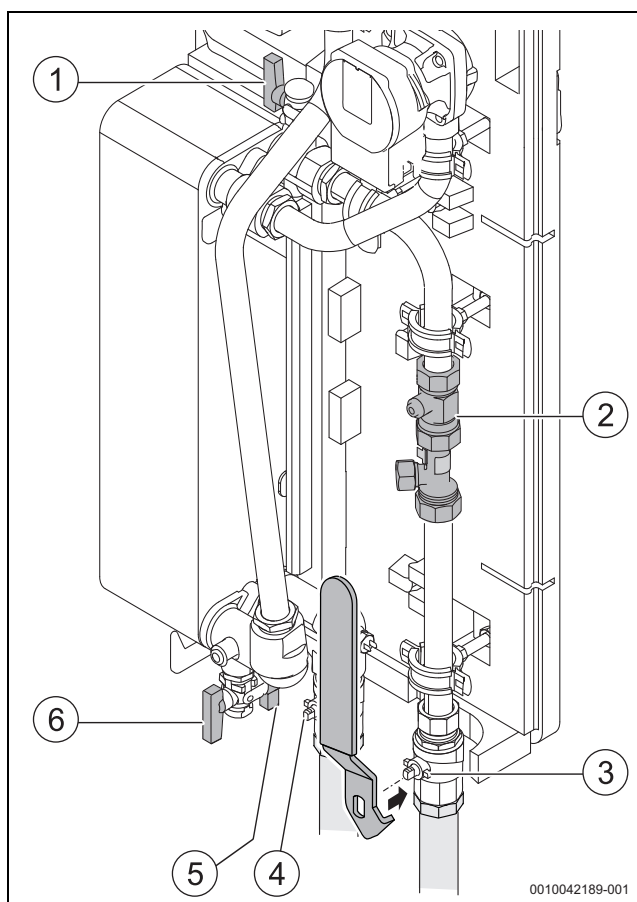
Bild 67 Volumenstromfühler wechseln
