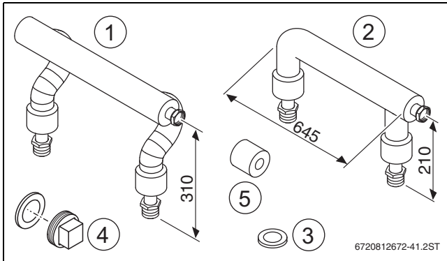
Bild 30 Lieferumfang Verrohrungssatz
