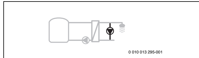
Bild 41 Zirkulation
