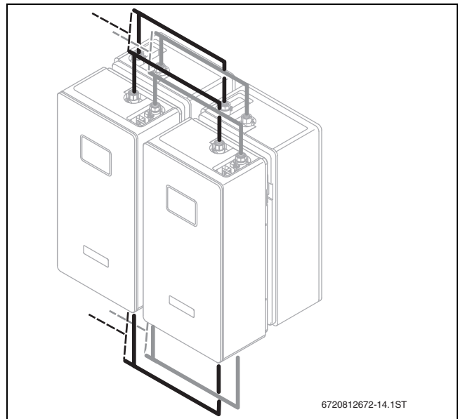
Bild 29 Beispiel: FS160S/3E mit 2 Verrohrungssätzen (alternativ: 4 Stationen bauseits in einer Reihe verbinden)
