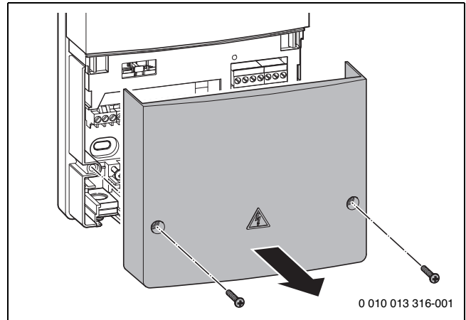
Bild 46 Modul öffnen
