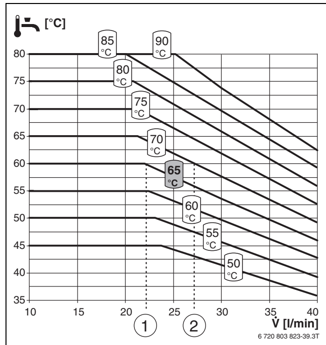
Bild 59 Temperaturverhalten Einzelstation FS27/3E
