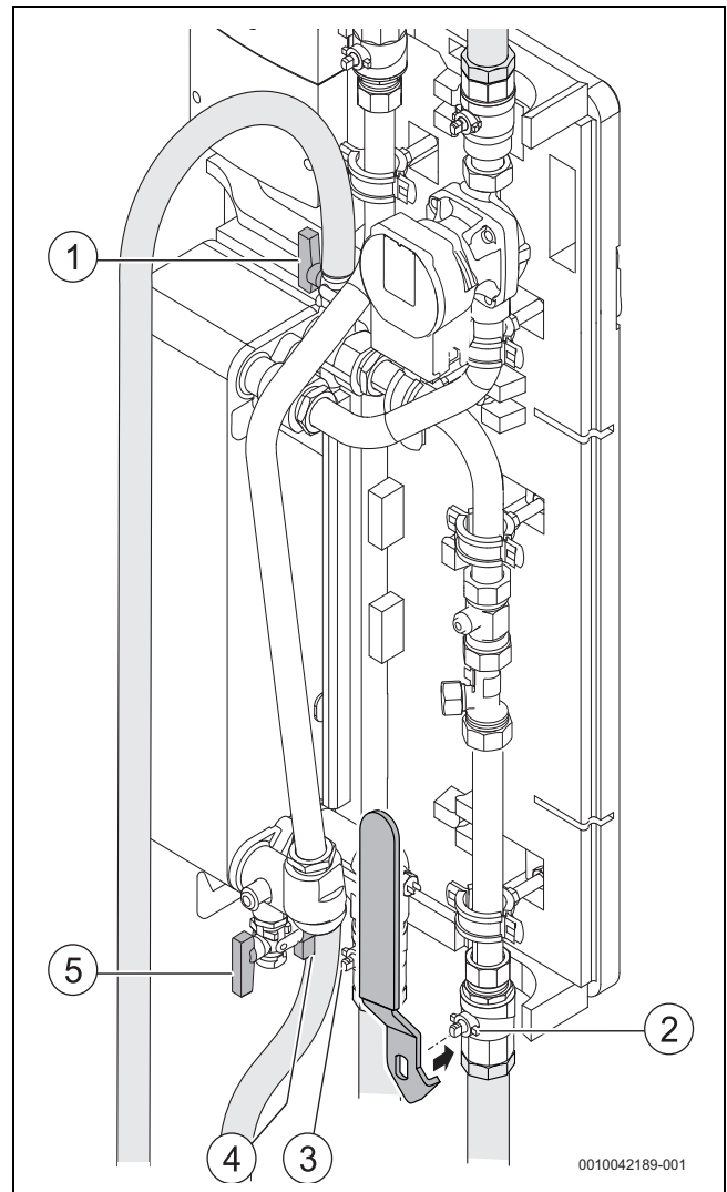
Bild 66 Wartung Frischwasserstation
