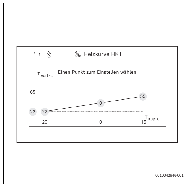
Bild 5 Startmenü Heizkurve
