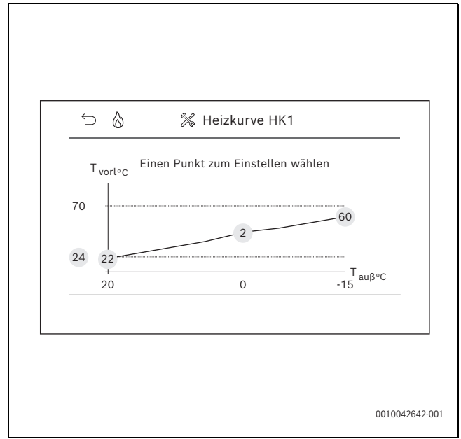
Bild 8 Komfortpunkt einstellen
