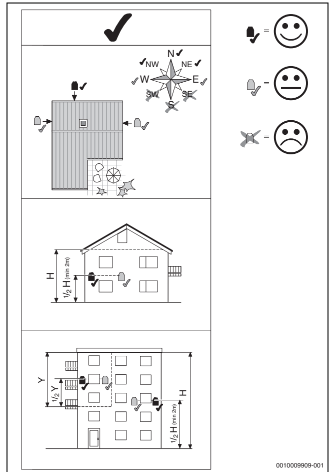
Bild 2 Geeigneter Installationsort des Außentemperaturfühlers
