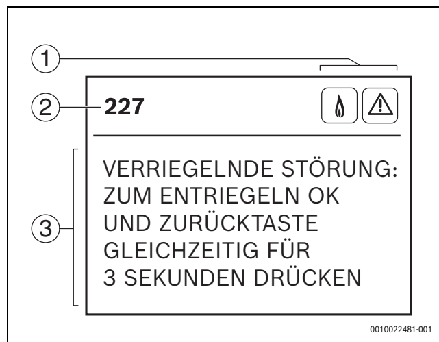
Bild 13 Störungsmenü (Beispiel)
