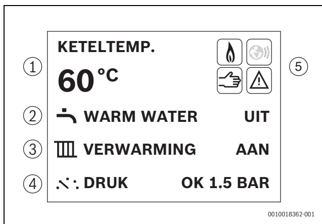
Bild 7 Standardanzeige
