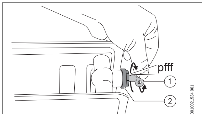
Bild 12 Heizkörper entlüften
