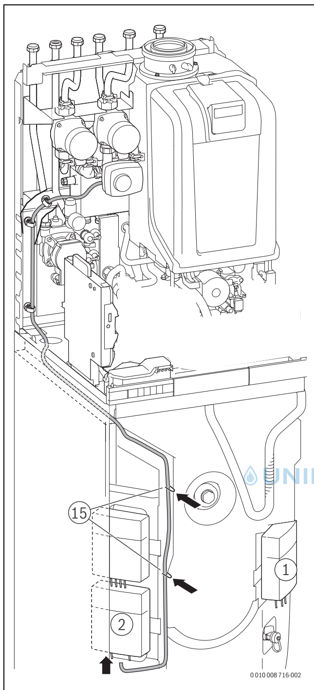
Bild 139 Anschluss Mischermotor
