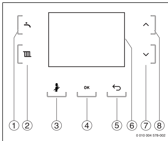
Bild 196 Bedienfeld
