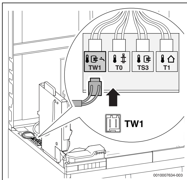
Bild 60 Speichertemperaturfühler anschließen
