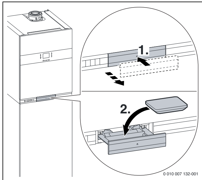
Bild 185 Heizungsregler einstecken
