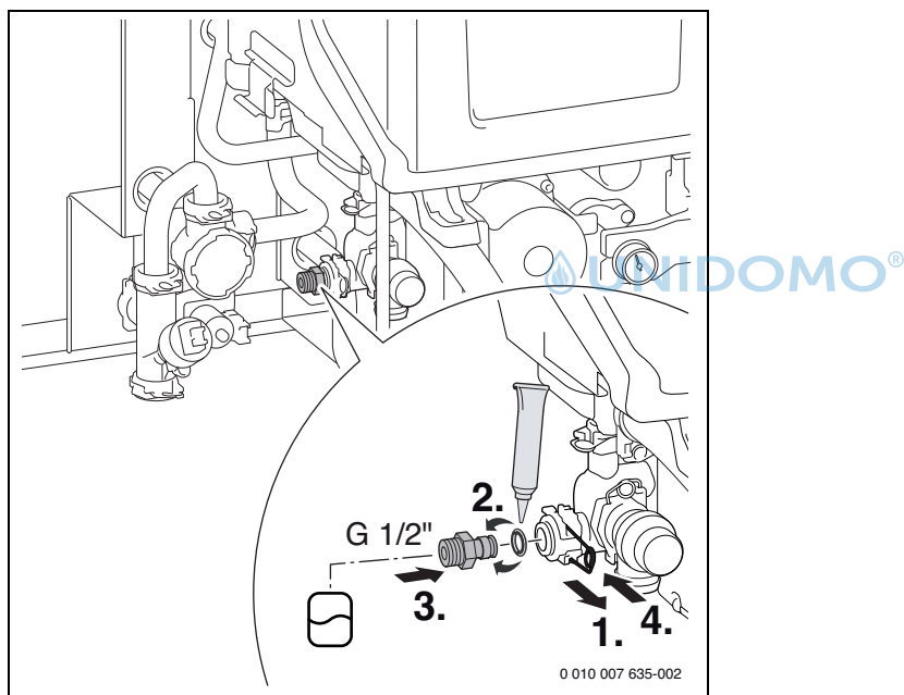
Bild 115 Verbindungsstück für den bauseitigen Anschluss eines externen Ausdehnungsgefäßes montieren
