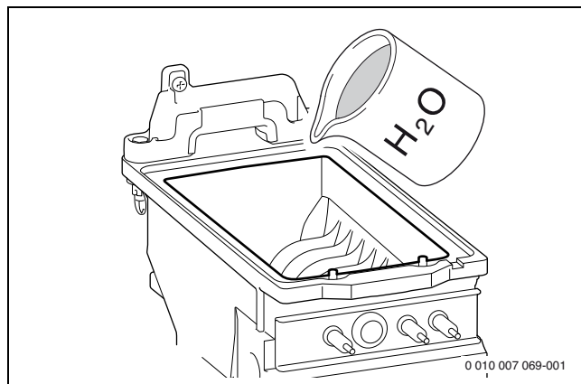
Bild 212 Spülen
