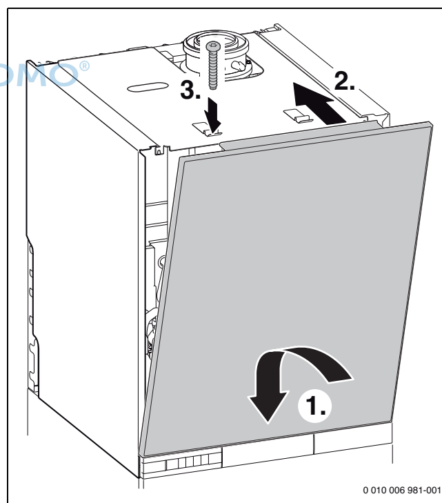
Bild 193 Vordere Verkleidung einhängen und mit Schraube aus Lieferumfang sichern
