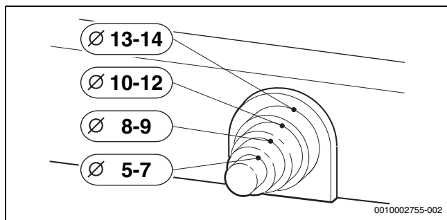
Bild 140 Zugentlastung Kabel Mischermotor anpassen
