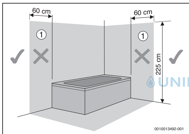
Bild 177 Schutzbereiche
