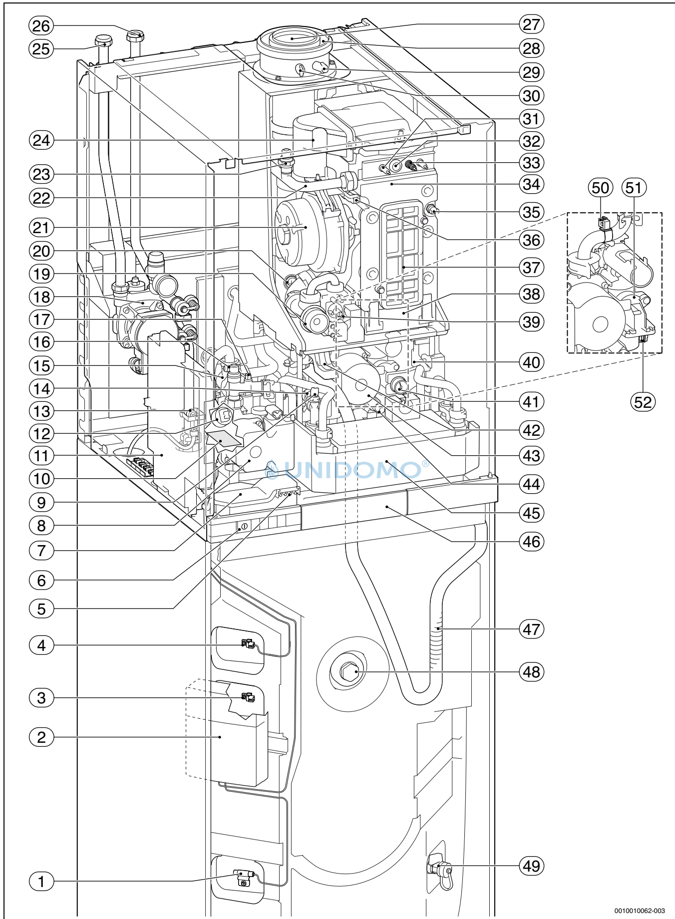
Bild 12 GB192... iT210...-Geräte
