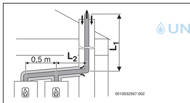
Bild 38 Kaskade mit 2 Geräten:
