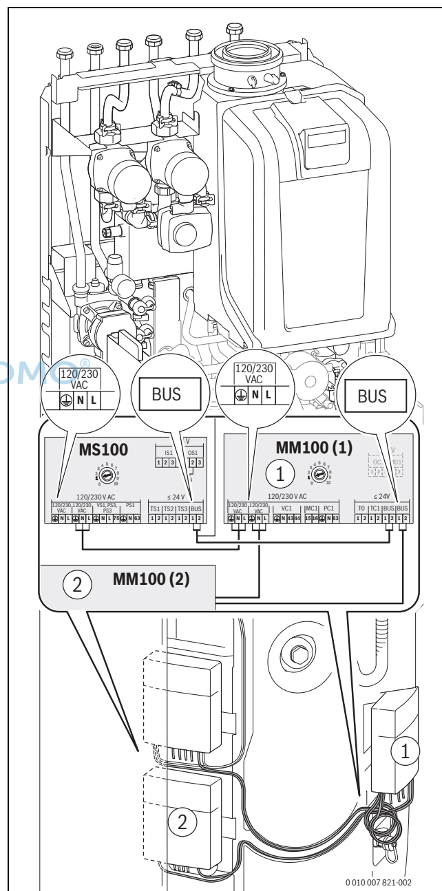
Bild 142 Anschluss am Modul MS100 und am Modul MM100 durchschleifen
