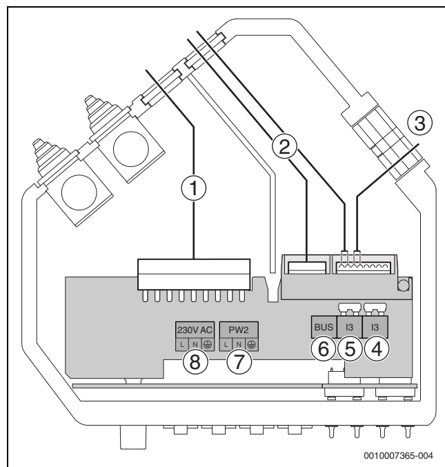
Bild 180 Anschlussbox
