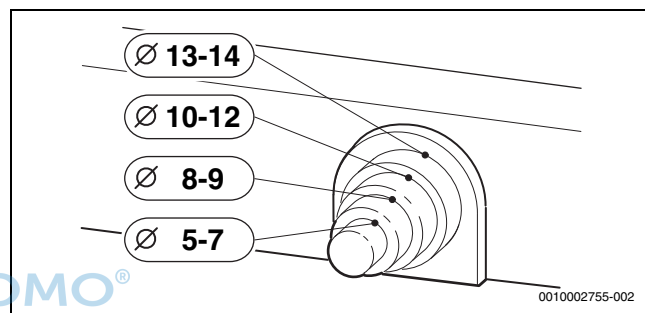
Bild 179 Zugentlastung an Kabeldurchmesser anpassen
