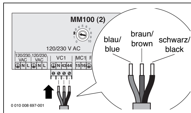
Bild 141 Anschluss Kabel Mischermotor am Modul MM100 [2]
