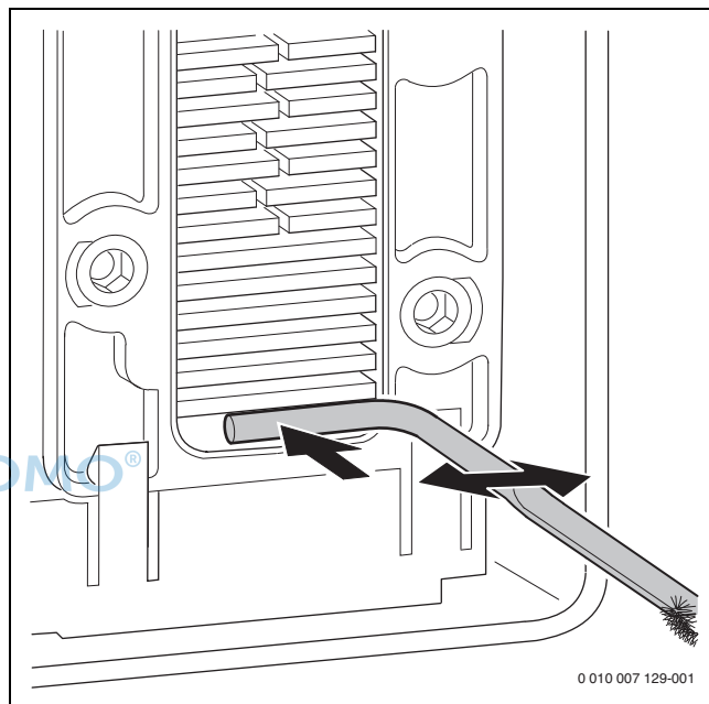
Bild 213 Kondensatwanne reinigen
