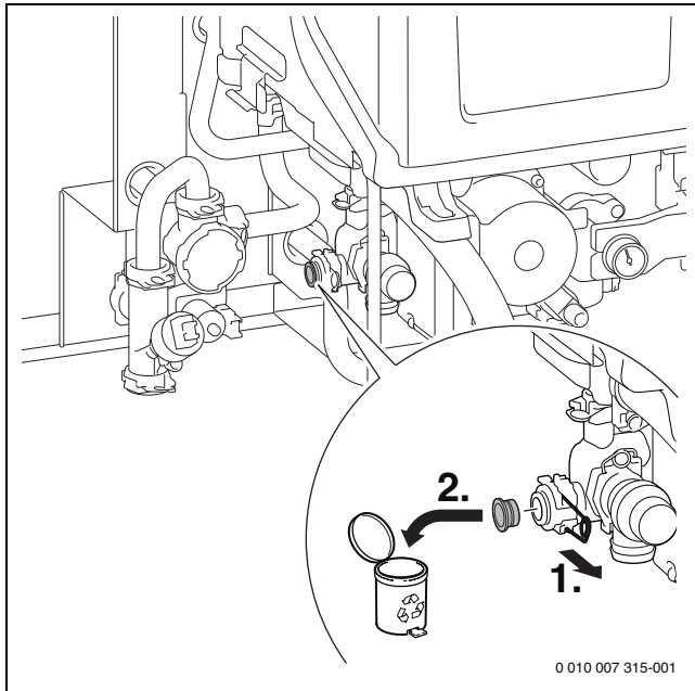
Bild 143 Stopfen entfernen
