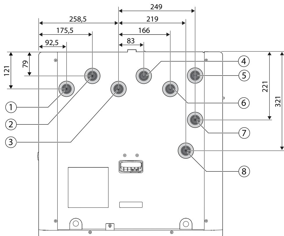
Bild 6 Ansicht von oben: Positionen der Anschlüsse
