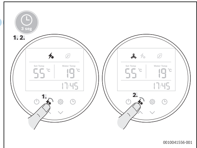
Bild 23 Einstellung Betriebsart "Nur elektrischer Zuheizter"
