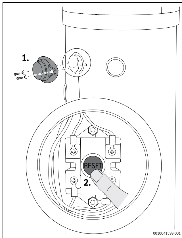
Bild 31 Thermostat-Reset
