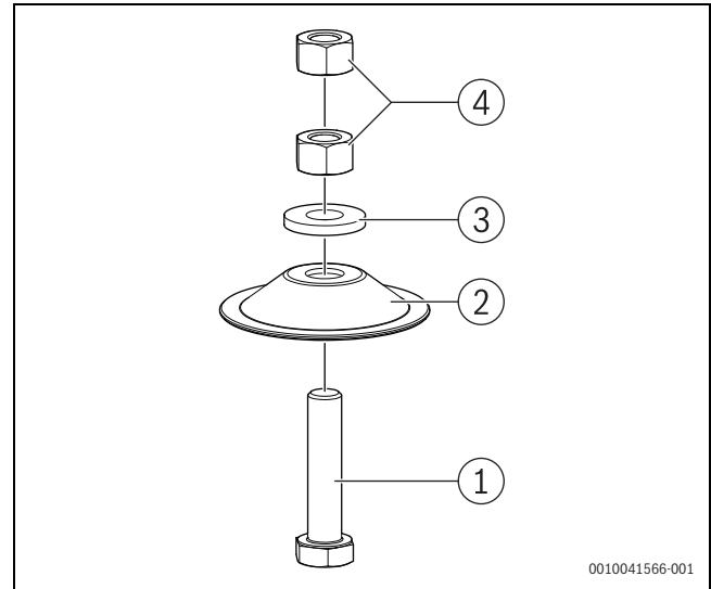
Bild 7 Zusammenbau der Stellfüße
