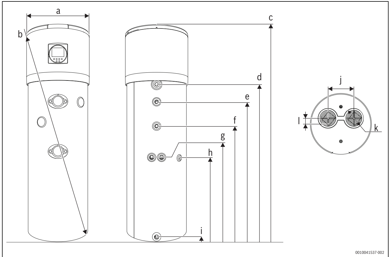
Bild 2 Geräteabmessungen
