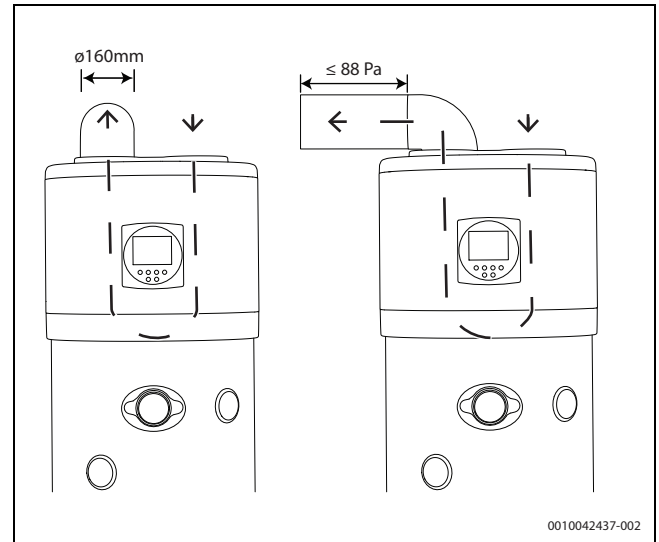
Bild 10 Einfache Luftleitung
