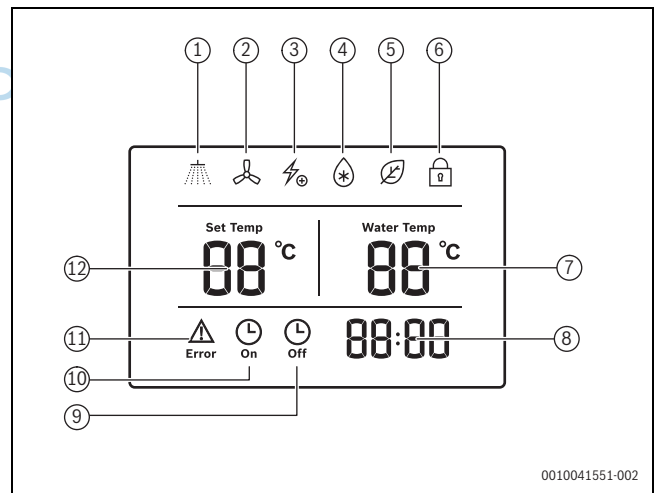
Bild 14 Bedienfeld - Display-Symbole
