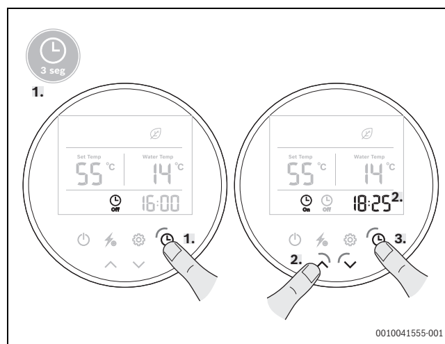
Bild 19 Timer-Einstellung
