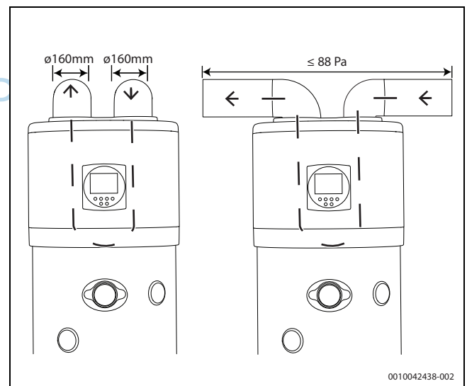
Bild 11 Zweite Luftleitung
