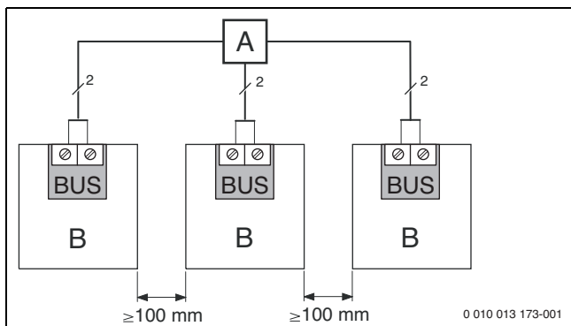
Bild 15 Verteilerdose anschließen
