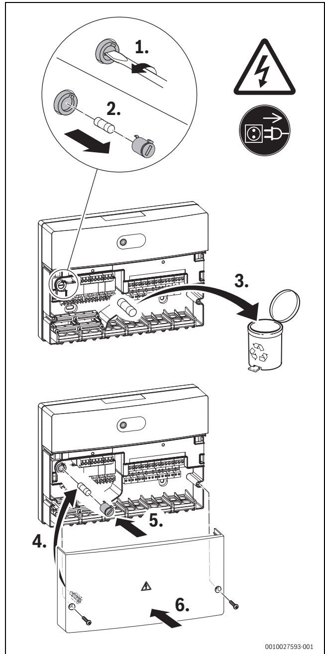
Bild 26 Sicherung tauschen
