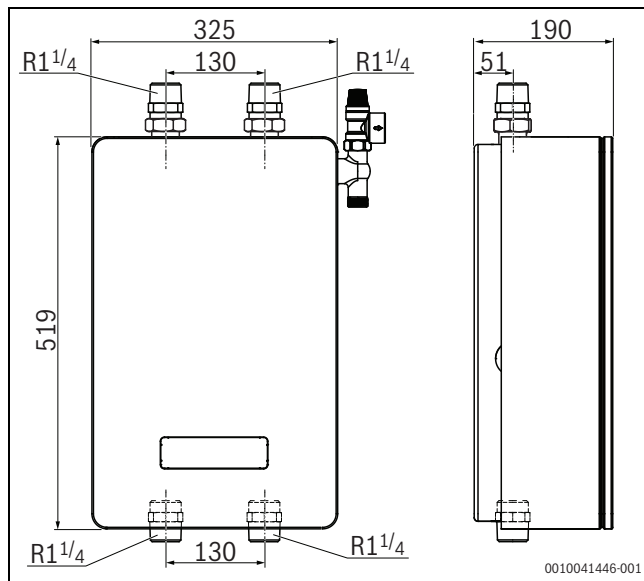
Bild 35 Abmessungen
