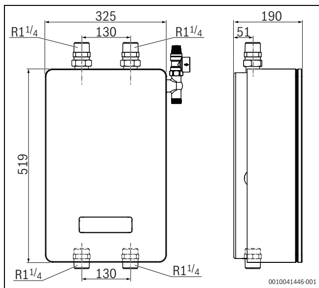
Bild 35 Abmessungen
