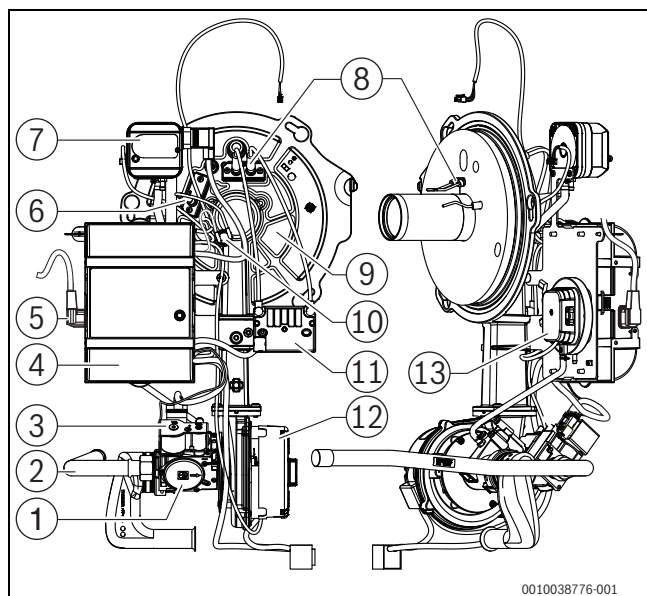
Bild 58 Vorderansicht/Rückansicht perspektivisch
