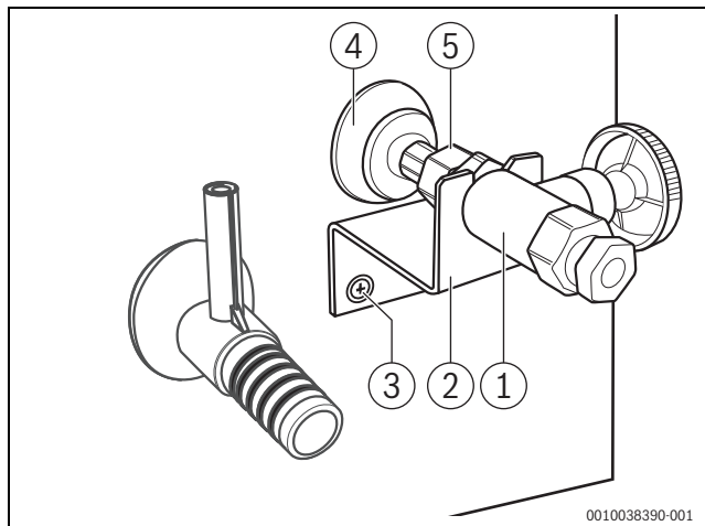
Bild 9 Öl-Absperrventil, Kesselrückseite
