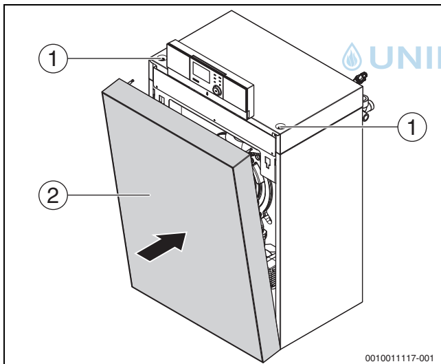
Bild 33 Kesselvorderwand montieren
