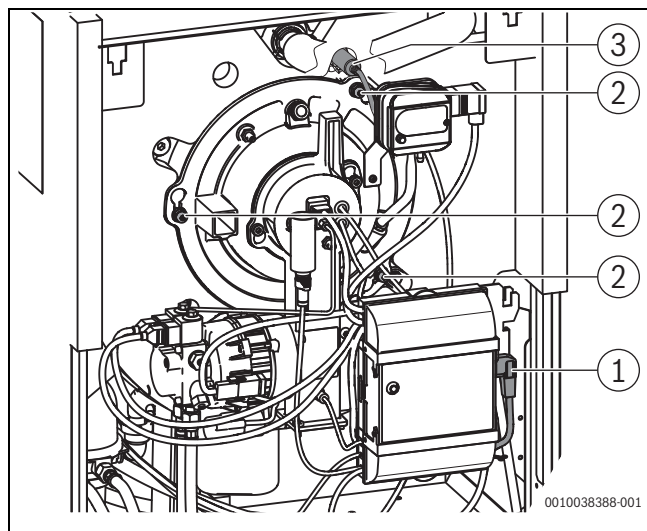
Bild 7 Ölbrenner ausbauen
