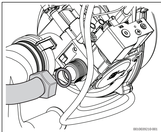
► Mitgelieferte Dichtung (im Zubehör-Set) in Schraubenverbindung des Gasrohres an der Gasarmatur einlegen und Überwurfmutter mit einem Drehmoment von 50 Nm anziehen (→ Bild 17). Dabei darauf achten, dass die Durchführungstülle des Gasrohres an der Rückwand gleichmäßig am Rohr anliegt und keine mechanischen Spannungen entstehen.
