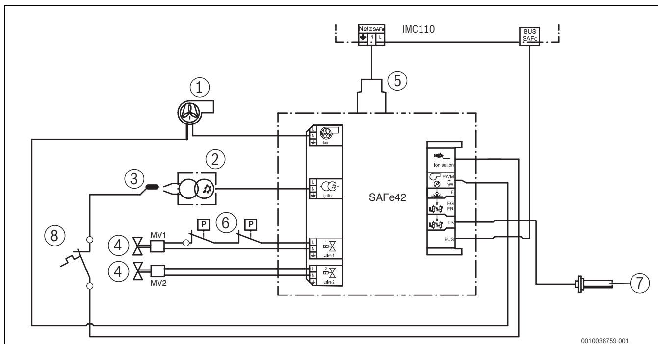
Bild 57 Anschlussplan Feuerungsautomat
