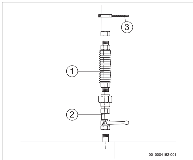
Bild 19 Gasanschluss herstellen
