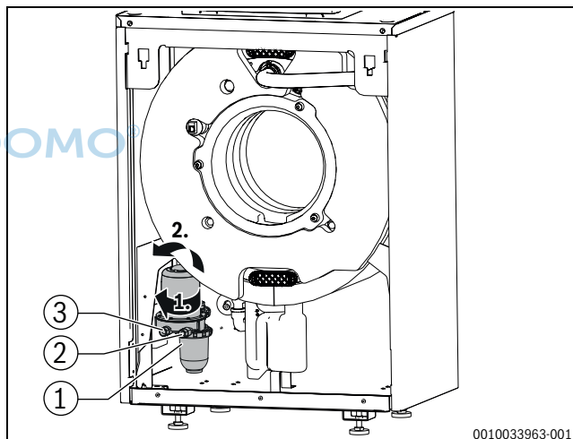
Bild 10 Ölfilter demontieren
