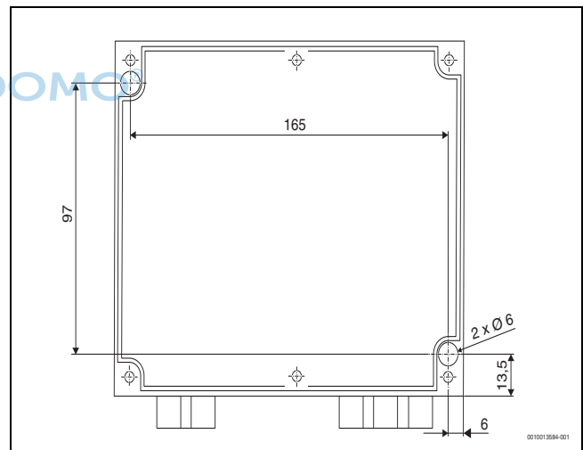
Bild 1 Befestigung des Moduls an der Wand
