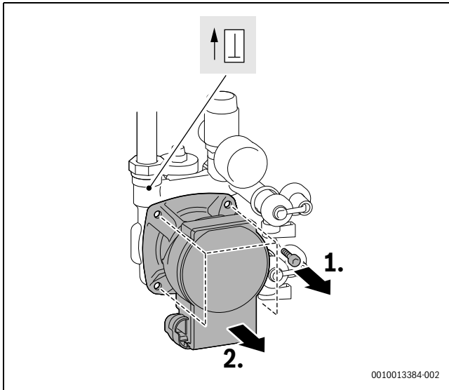
Bild 184 Solarpumpe ausbauen
