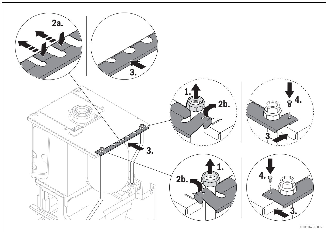
Bild 81 Rohrhalter am Oberteil der Geräteverkleidung befestigen
