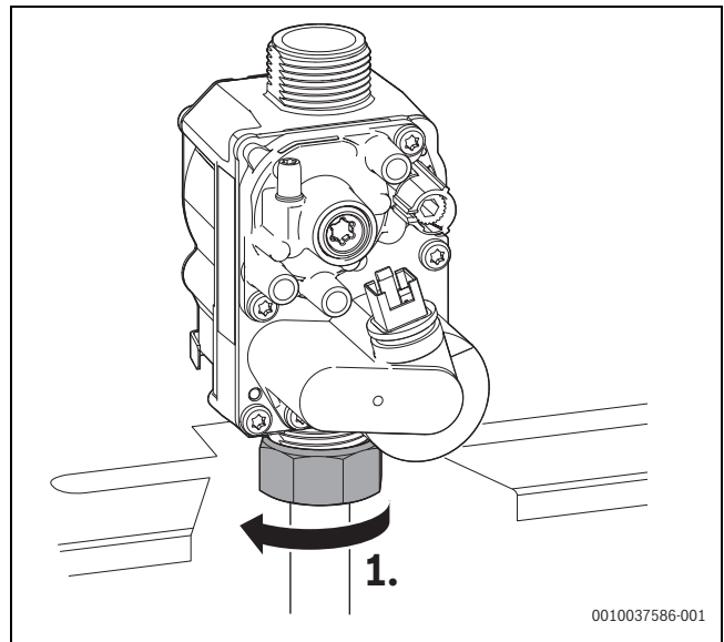
Bild 162 Überwurfmutter lösen
