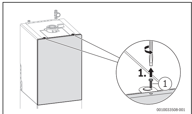
Bild 133 Sicherungsschraube lösen
