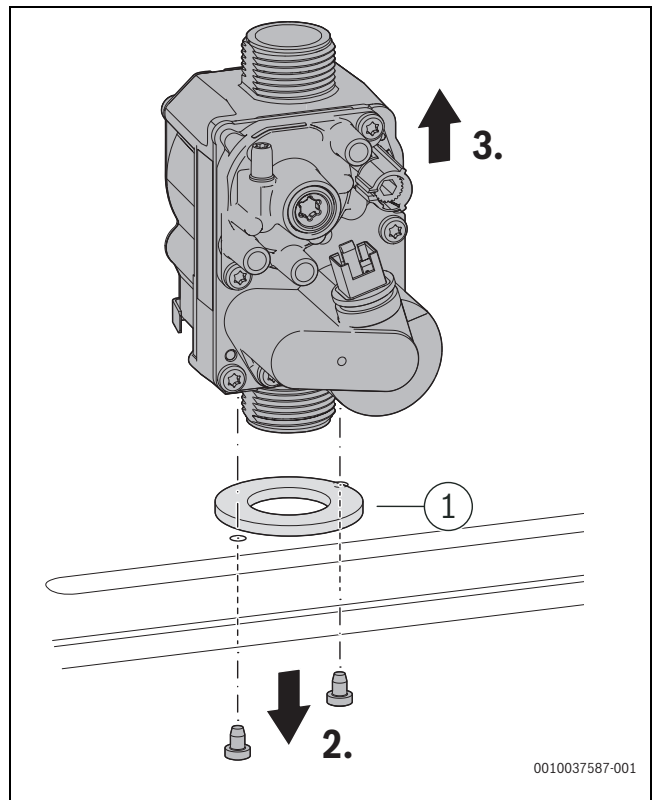
Bild 163 Gasarmatur ausbauen
