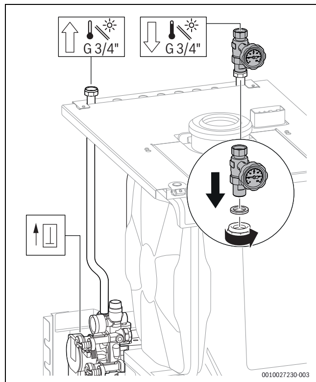
Bild 83 Wartungshahn am Solar-Vorlaufrohr anschließen
