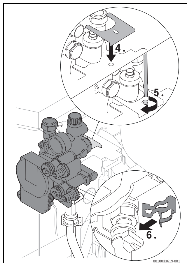
Bild 73 Solarstation befestigen
