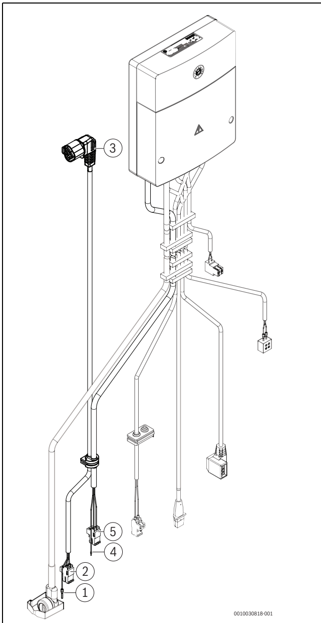
Bild 107 Spannungsversorgung Schichtladepumpe und Solarmodul
