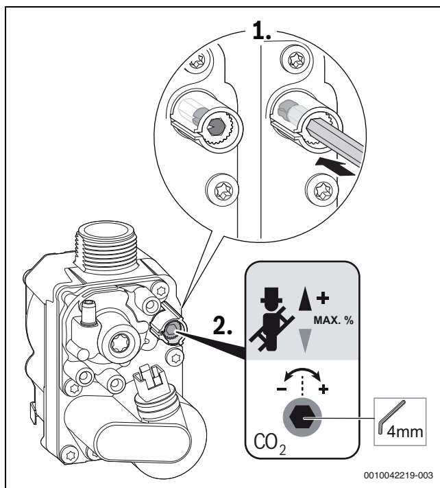
Bild 128 CO 2 /O 2 -Gehalt bei maximaler Nennwärmeleistung einstellen
