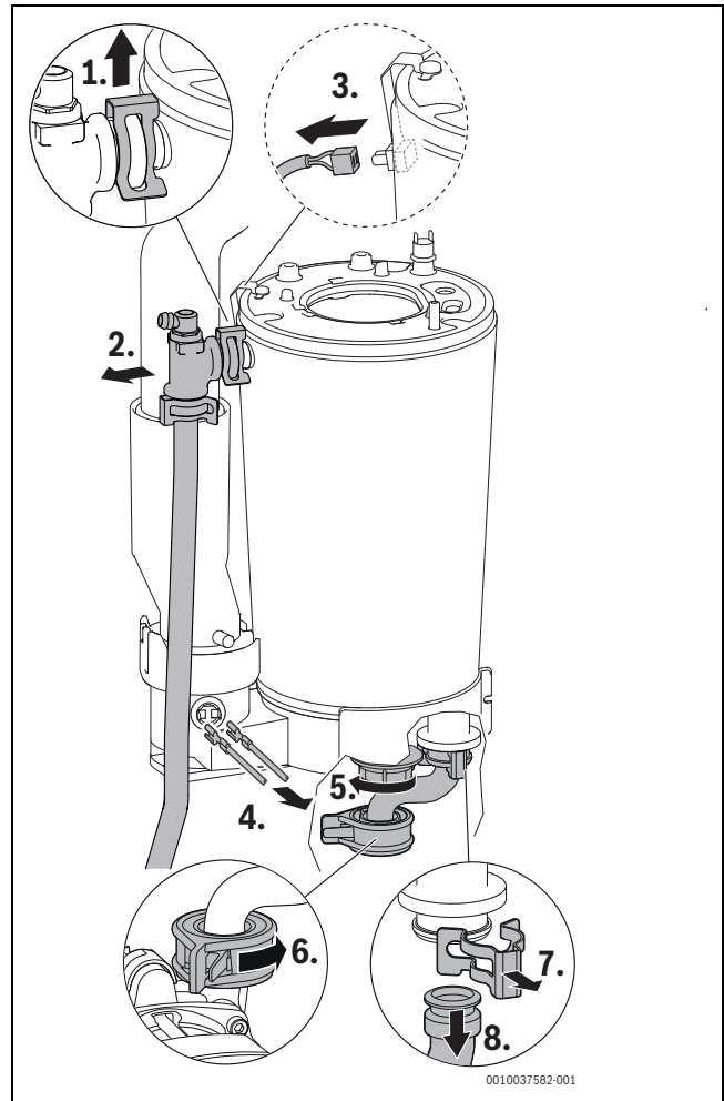
Bild 154 Vorlaufrohr lösen, Kabel abziehen und Rücklaufrohr lösen
