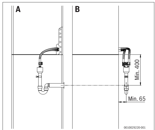
Bild 15 A: Ansicht von der rechten Seite (Maße in mm) B: Ansicht von vorn (Maße in mm)
