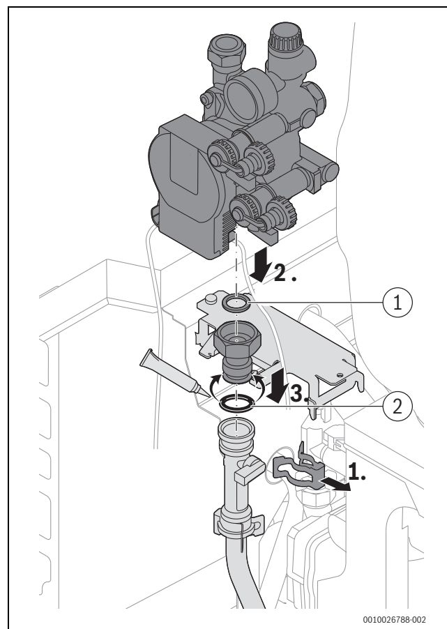
Bild 72 Solarstation einsetzen
