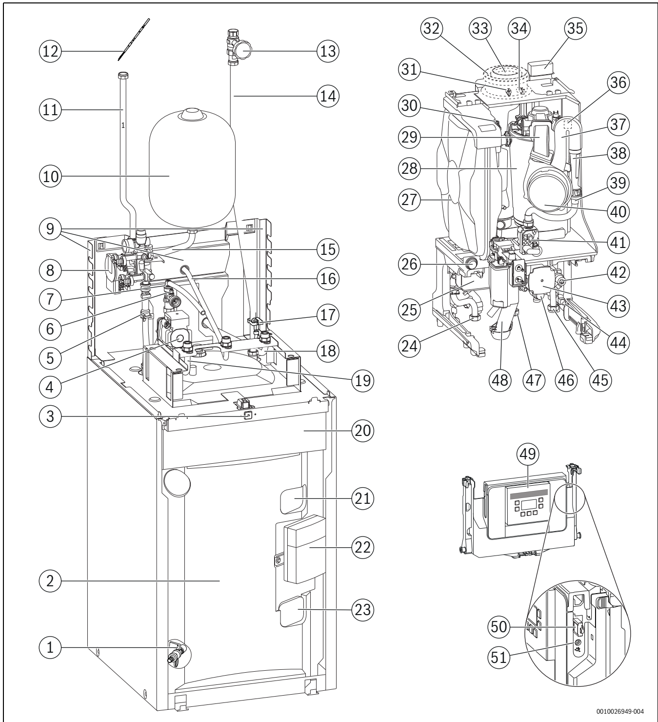
Bild 4 Produktübersicht
