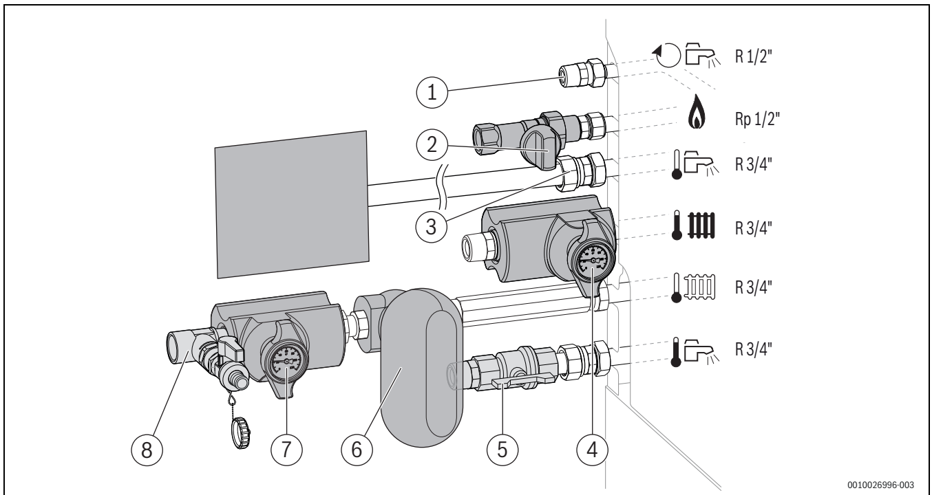
Bild 94 Armaturen-Set Zubehör CS 28-1 – Beispiel: Anschlüsse horizontal auf der linken Seite
