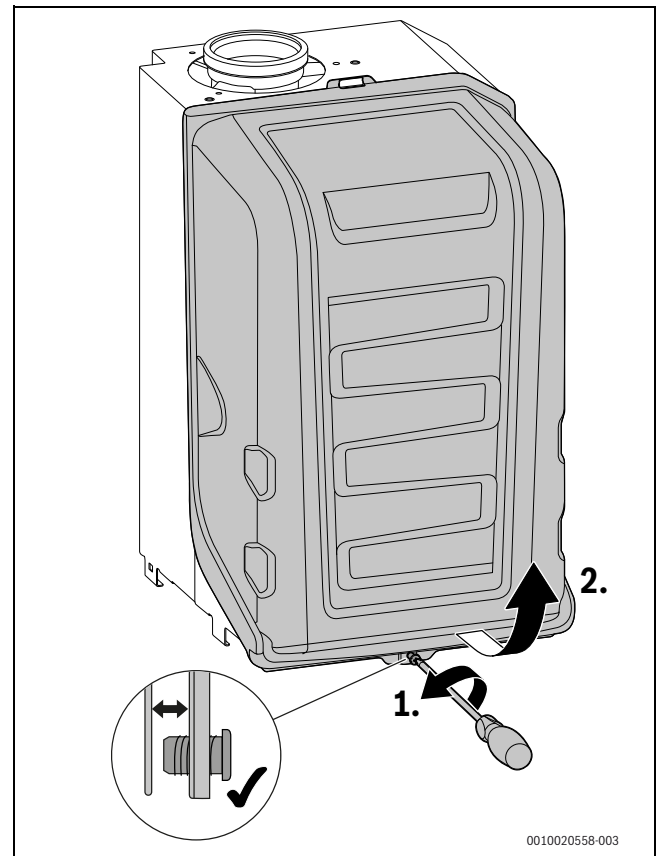
Bild 95 Brennerhaube abnehmen
