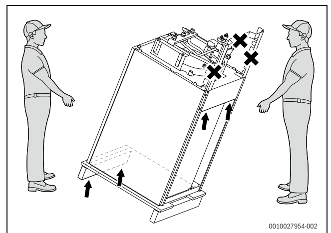
Bild 48 Transport des Speichers
