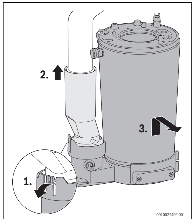
Bild 155 Wärmeblock ausbauen
