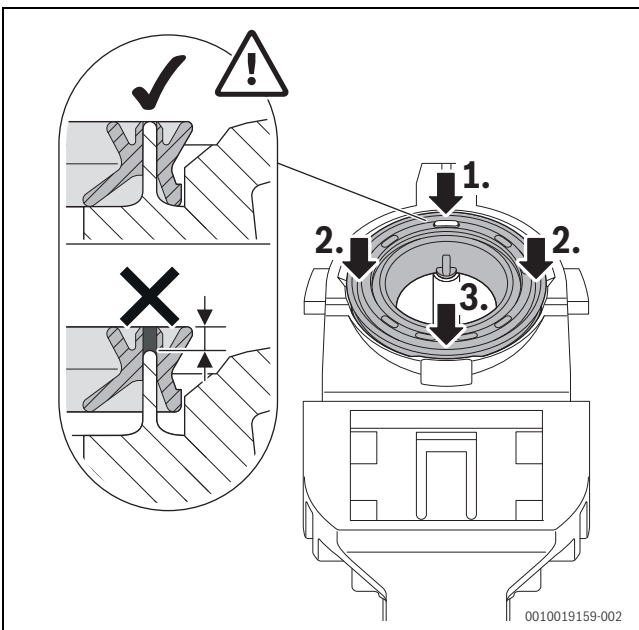
Bild 171 Dichtung andrücken
