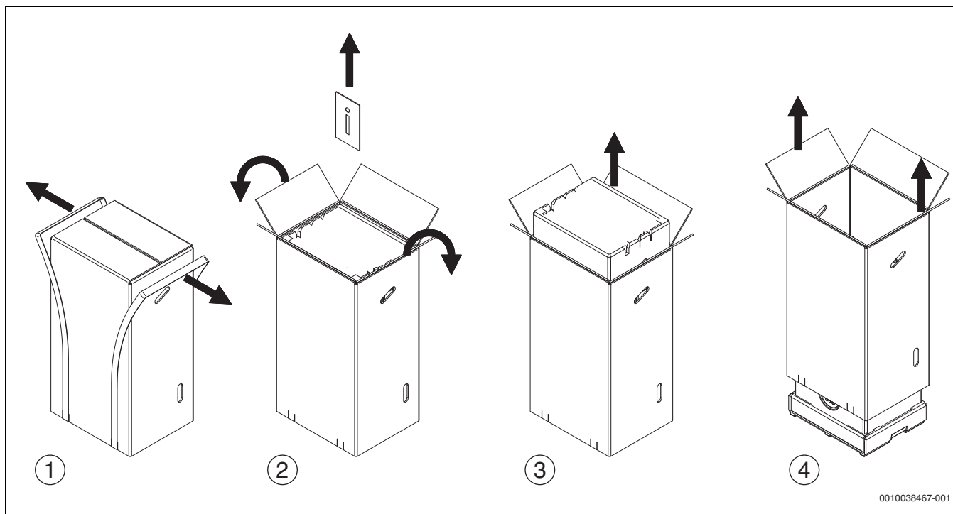
Bild 34 Auspackanweisung
