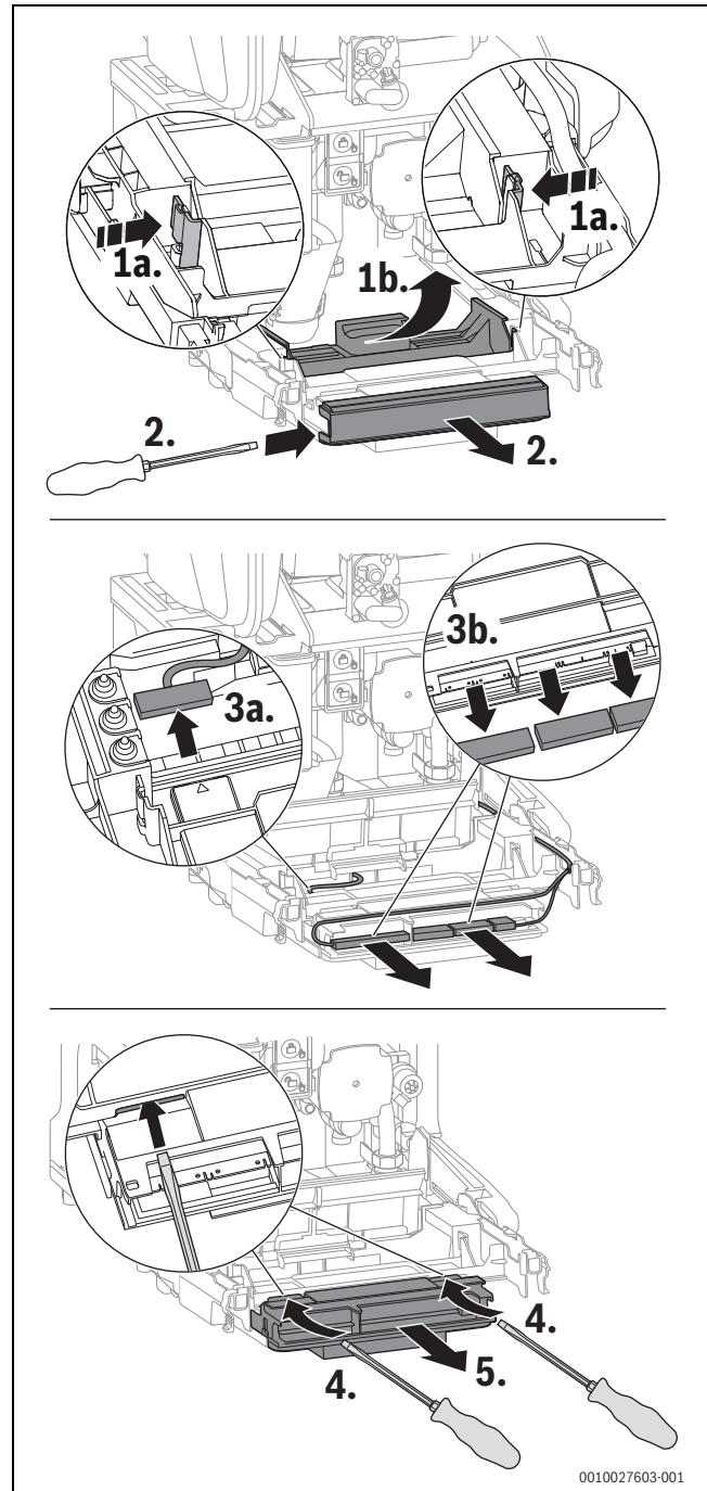
Bild 86 Steuergerät herausnehmen
