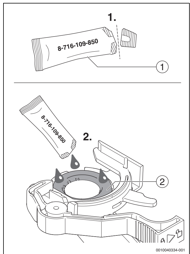
Bild 90 Dichtung fetten
