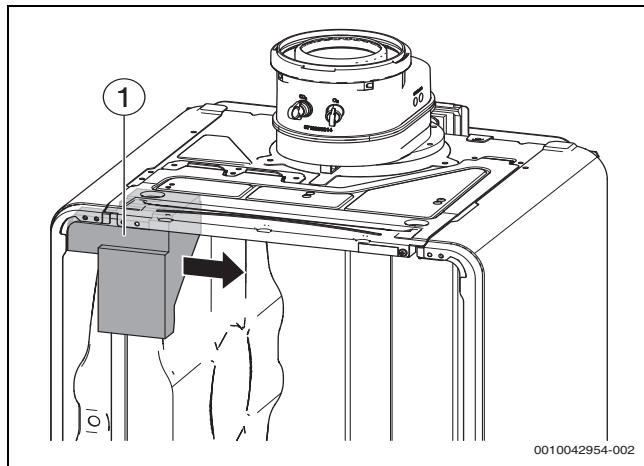
Bild 37 Stützschaum entfernen
