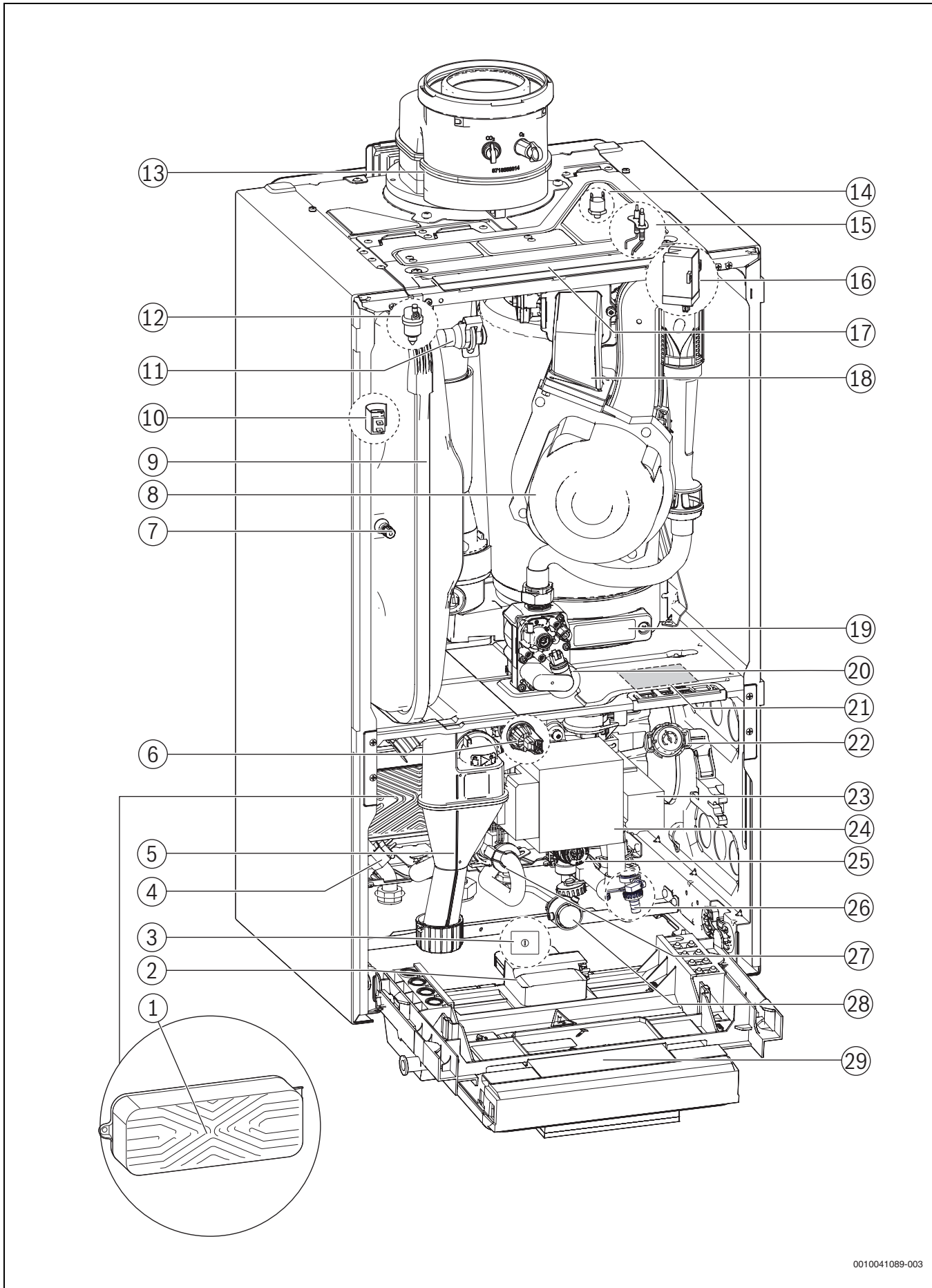
Bild 4 Produktübersicht
