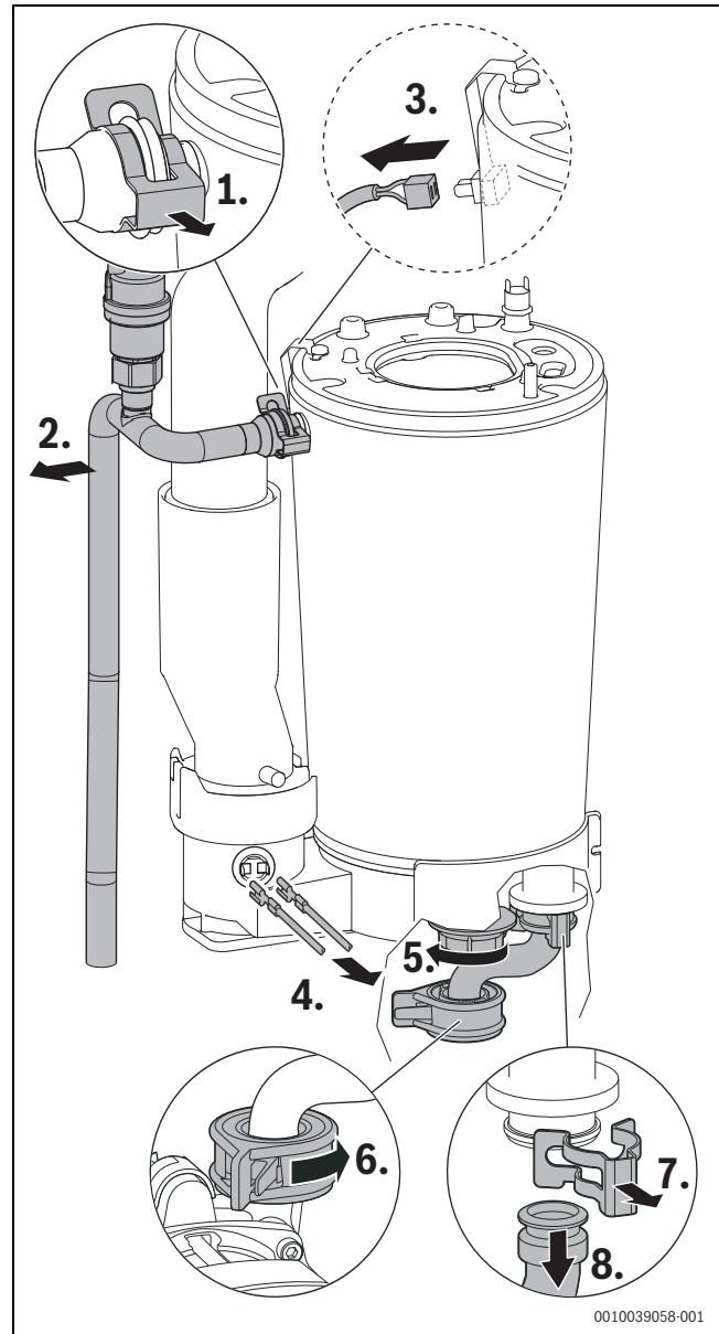
Bild 72 Vorlaufrohr lösen, Kabel abziehen und Rücklaufrohr lösen
