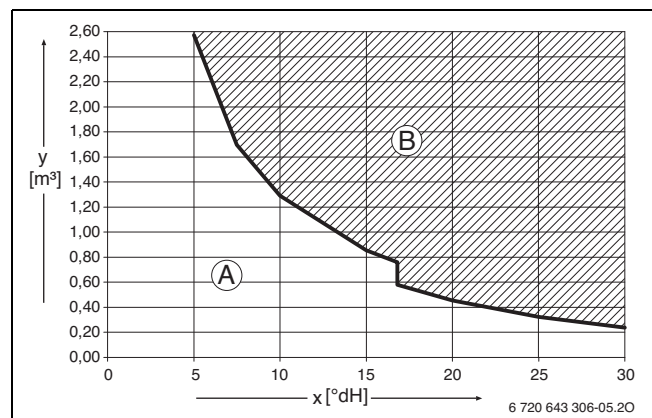
Bild 31 Anforderungen an Füll- und Ergänzungswasser Geräte &lt; 50 kW
