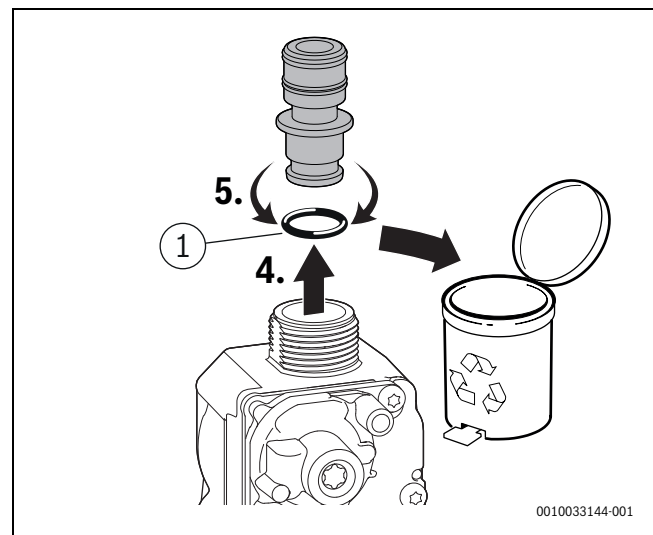
Bild 79 Gasschloss abnehmen
