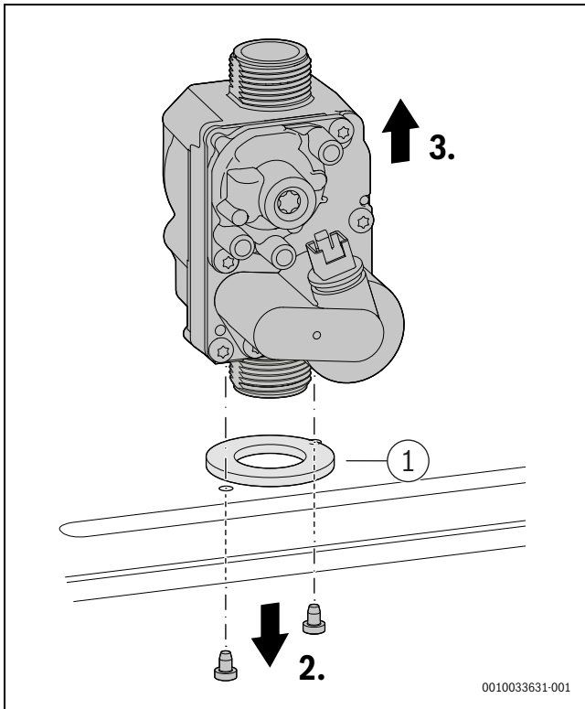
Bild 81 Gasarmatur ausbauen
