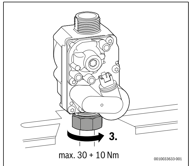
Bild 83 Anzugsdrehmoment beachten
