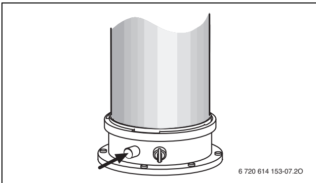
Bild 50 Abgasmessstutzen
