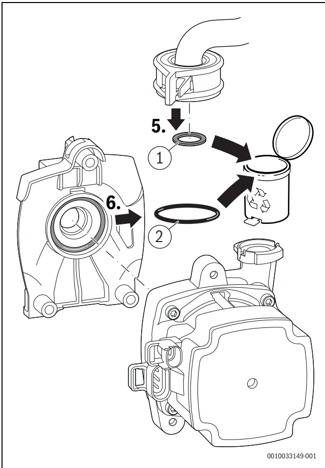
Bild 77 Dichtungen entsorgen
