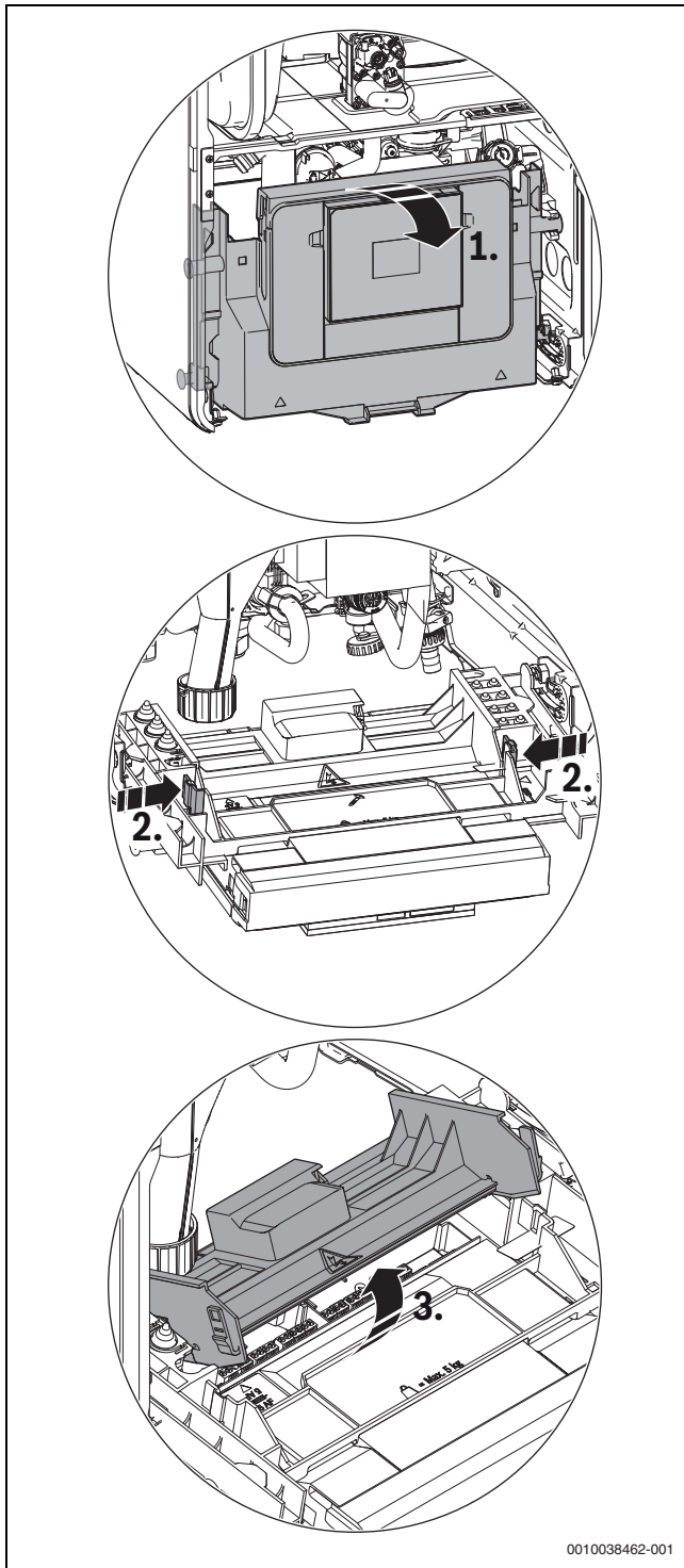
Bild 43 Abdeckung aufklappen
