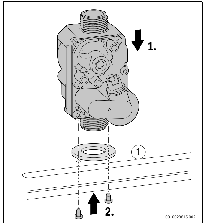
Bild 82 Gasarmatur einbauen
