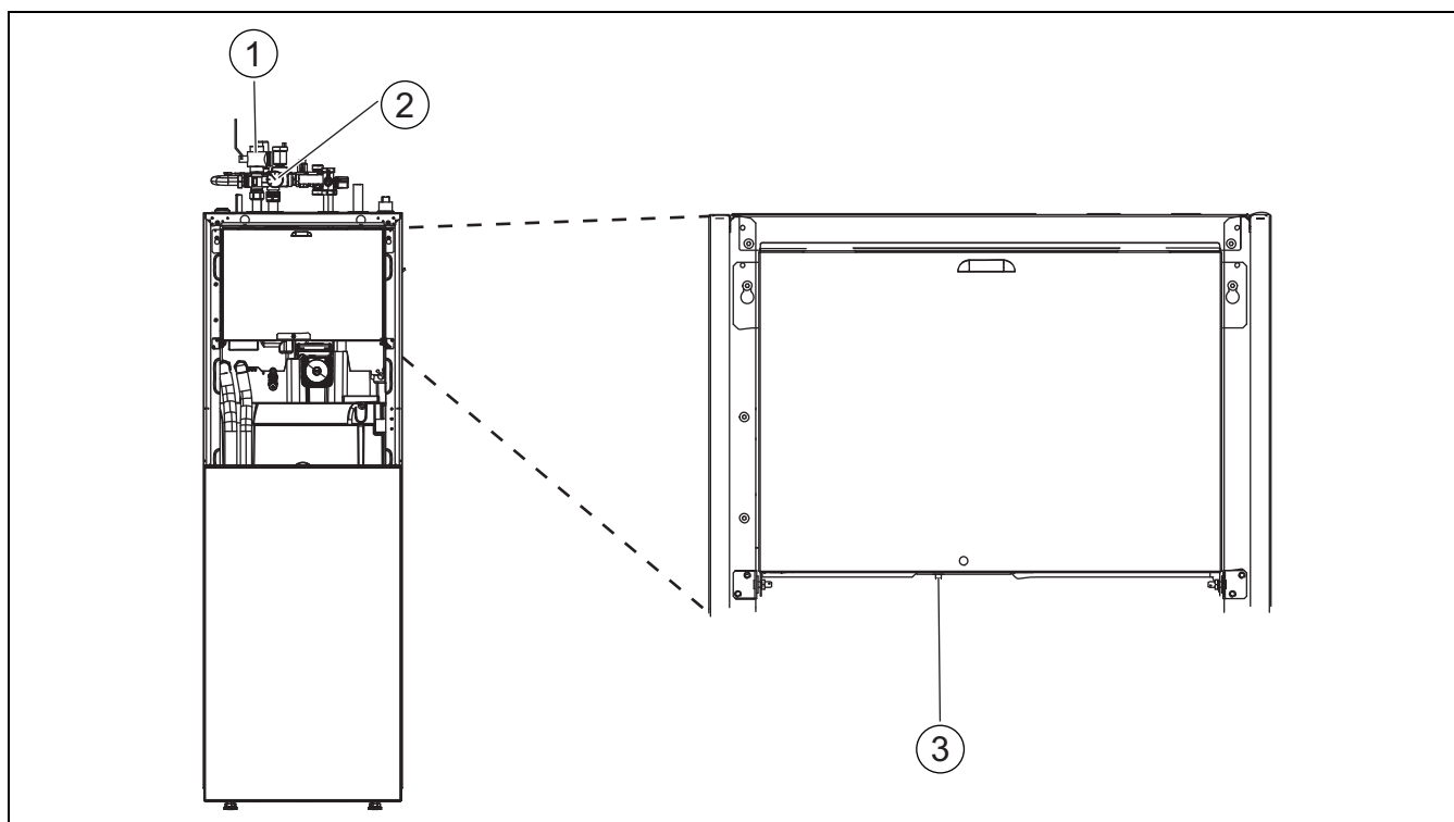
Bild 6 IDU-..iT / IDU-..iTS
