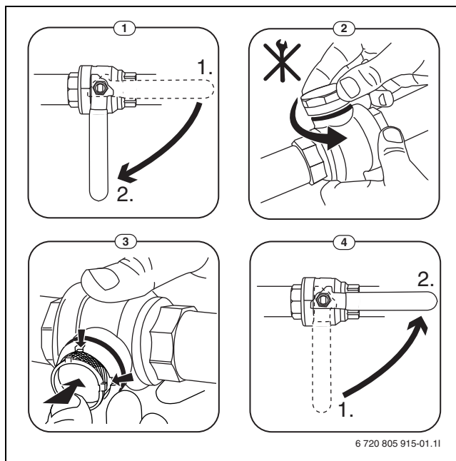
Bild 8 Siebreinigung
