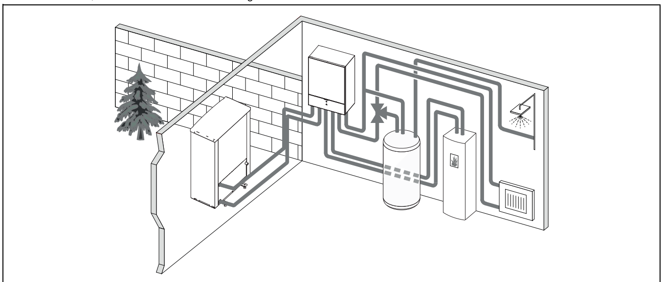
Bild 3 Wärmepumpe WLW196i.2 AR/IR, Inneneinheit IDU-..iB ohne elektrischen Zuheizter, externer Warmwasserspeicher und externer Zuheizter
