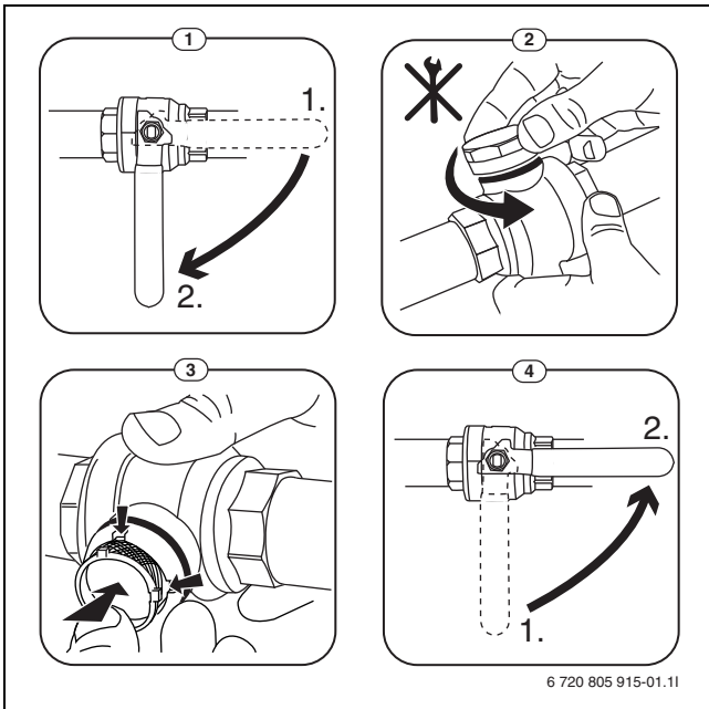
Bild 7 Siebreinigung
