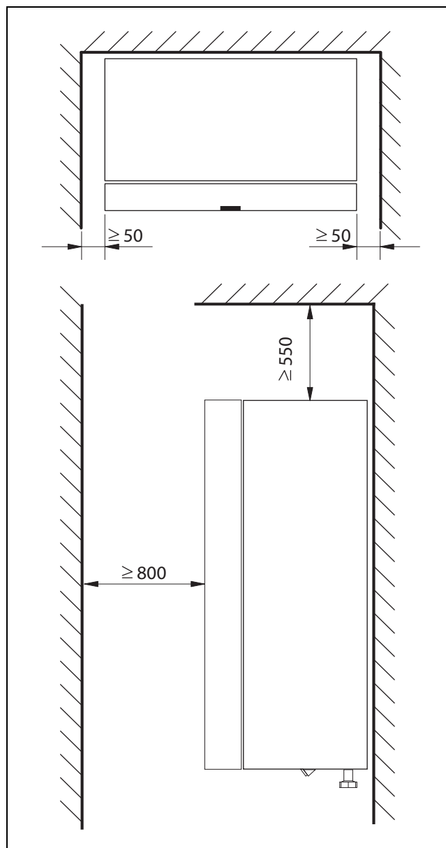
Bild 4 Mindestabstand (mm)
