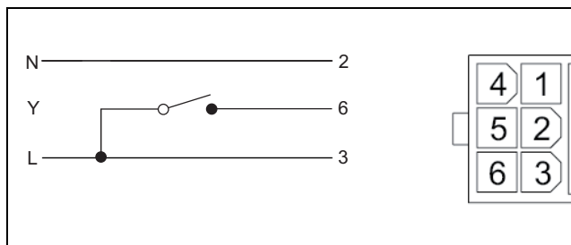
Bild 24 Molex-Stecker
