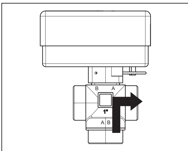
Bild 22 Kontakt geschlossen, Anschluss A offen
