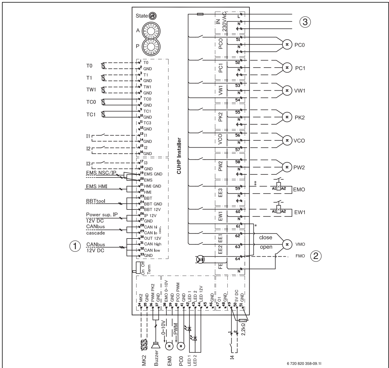
Bild 33 Schaltplan Installationsmodul für Inneneinheit mit Mischer für externen Zuheizer
