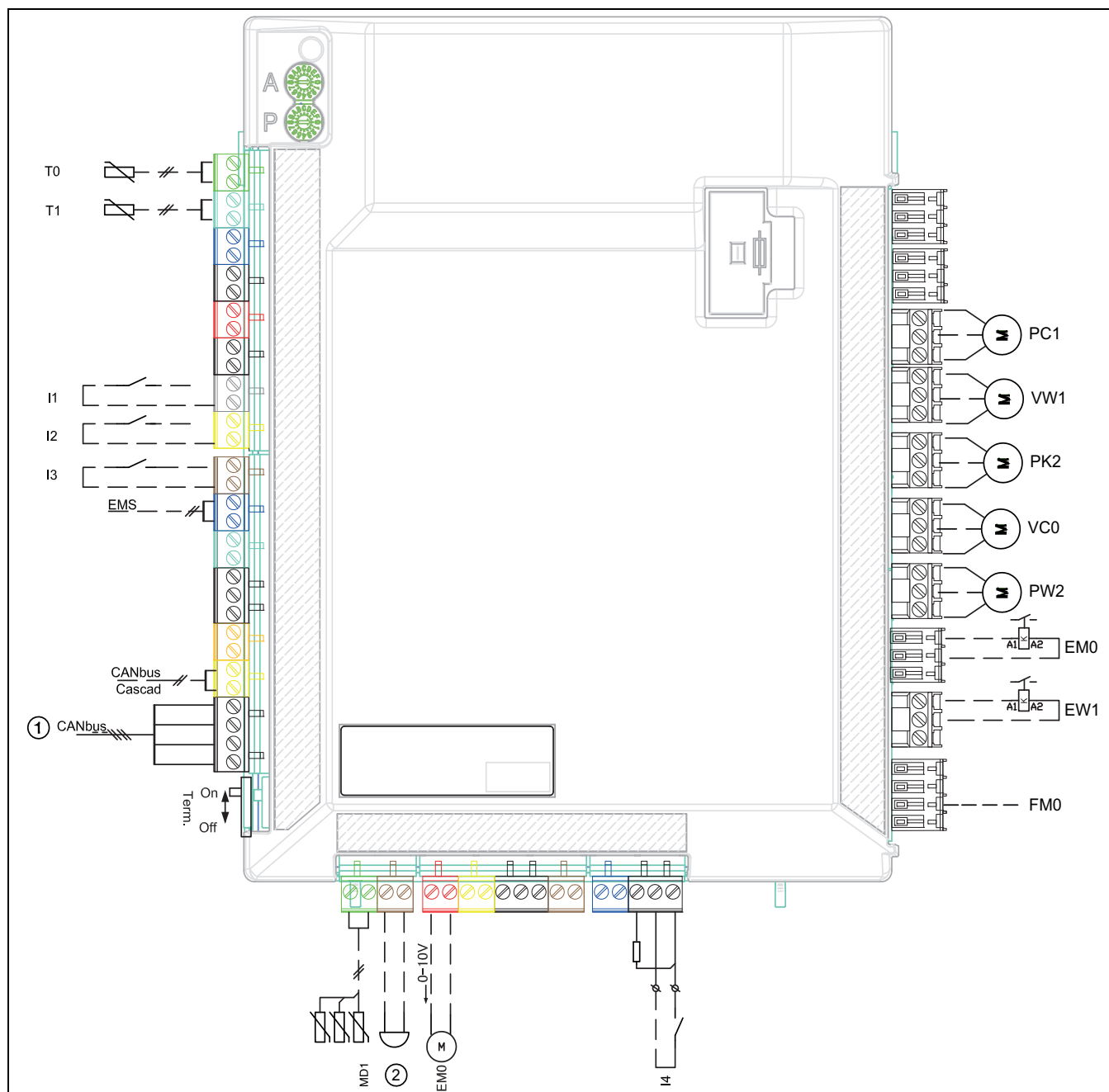
Bild 13 Anschlüsse Installationsmodul
