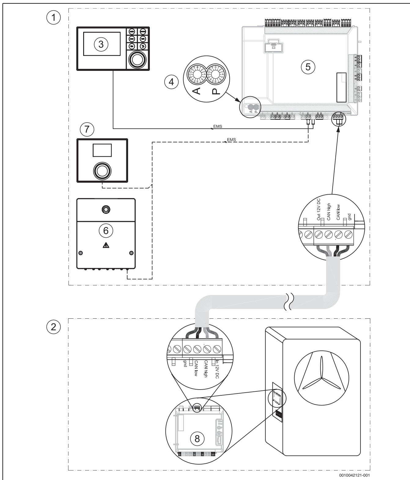
Bild 30 Inneneinheit mit Mischer für externen Zuheizer – Überblick CAN-/EMS-BUS
