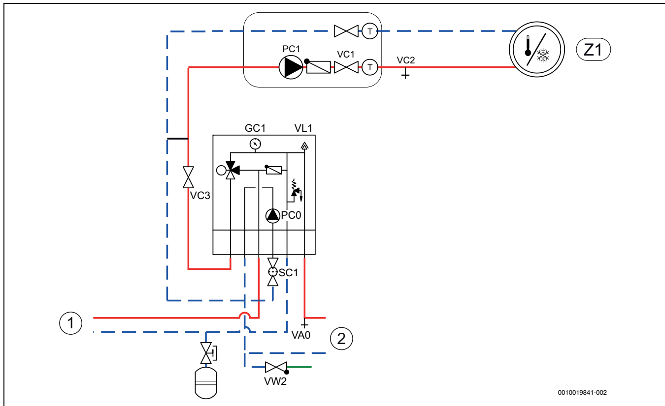
Bild 16 Inneneinheit mit externem Zuheizter und Heizsystem
