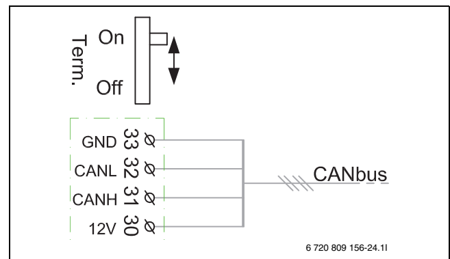
Bild 10 CAN-BUS-Terminierung
