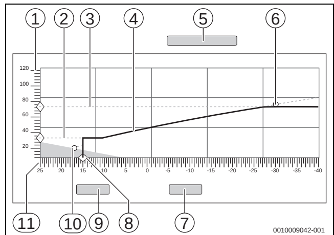
Bild 50 Heizkurven für die Heizsysteme „Heizkörper“ und „Fußboden“
