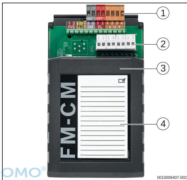
Bild 71 Funktionsmodul FM-CM
