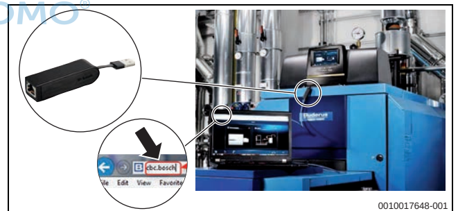
Bild 102 Servicetool Logamatic 5000 Adapter USB (Regelgerätseite) zu IP (PC-Seite: RJ45)
