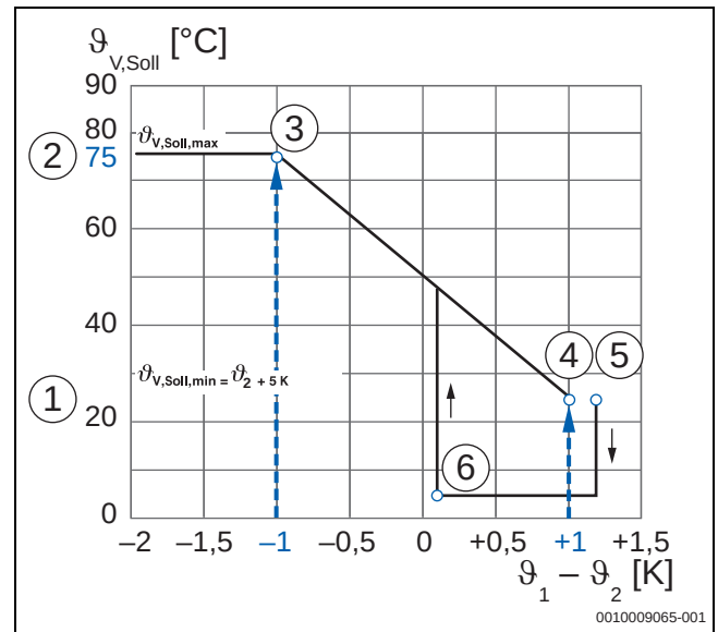
Bild 52 Heizkurve für das Heizsystem „Raumtemperaturgeführter Regler“
