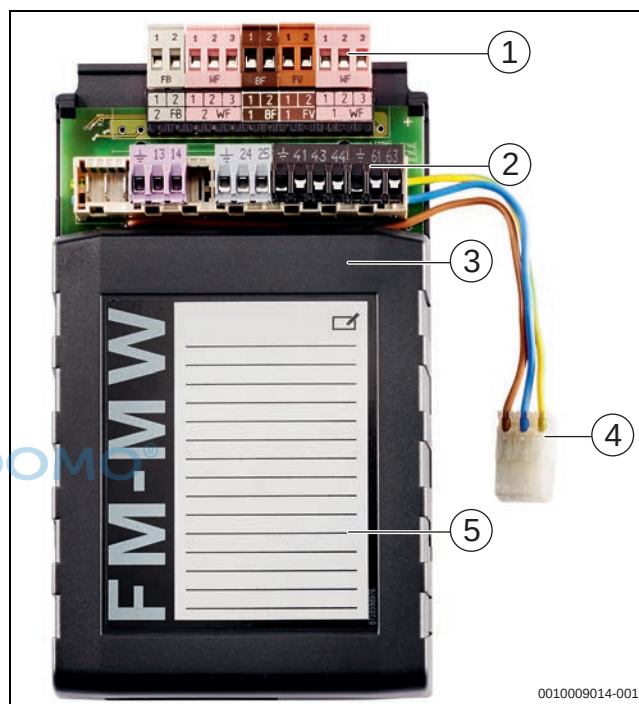
Bild 55 Funktionsmodul FM-MW
