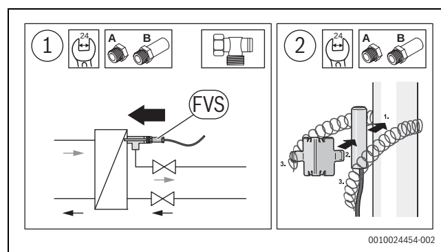
Bild 80 Fühlermontage am Wärmetauscher; Pos 1: optimiert, Pos 2: Standard Anlagefühler
