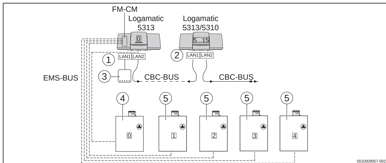
Bild 77 Kombinationsbeispiel der Regelgeräte des Systems Logamatic 5000 für eine 5-Wandheizgeräte-Kaskade mit Zuordnung des Heizkessels sowie der Adressen im CBC-BUS-Verbund
