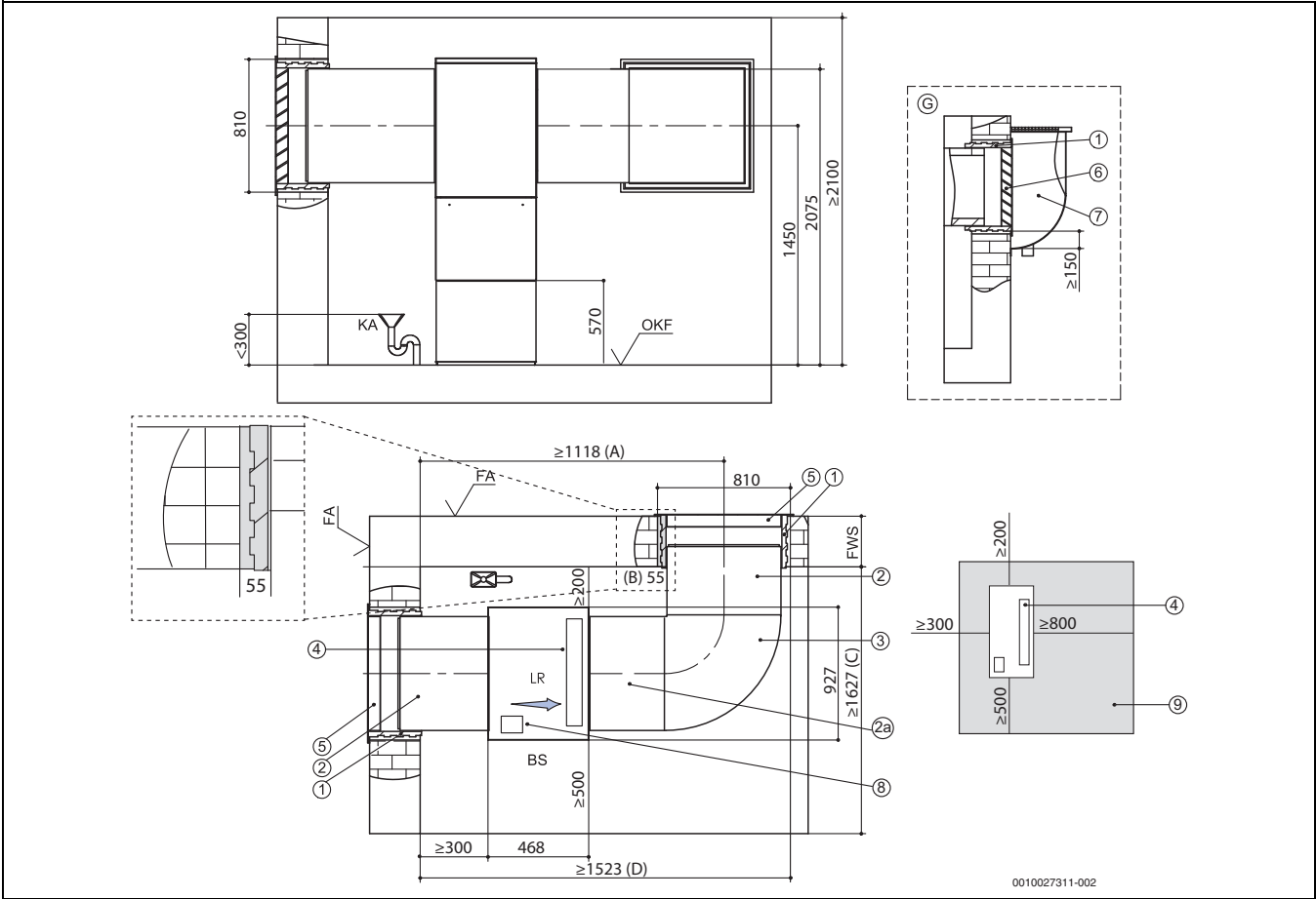
Bild 39 Kanalpläne Variante 1
