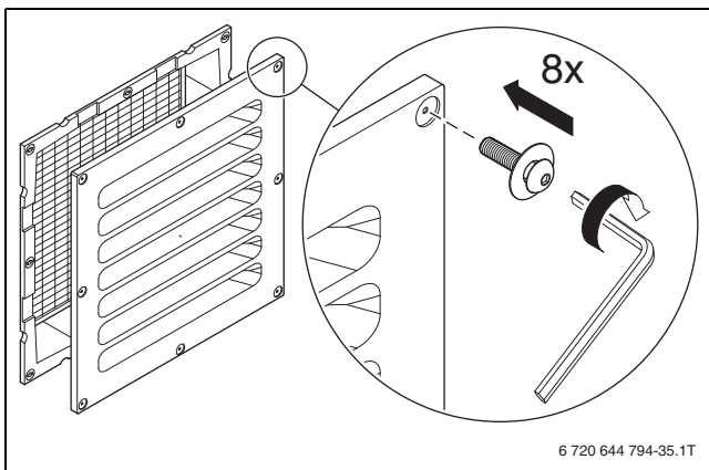
Bild 28 Wetterschutz-/Regenschutzgitter befestigen
