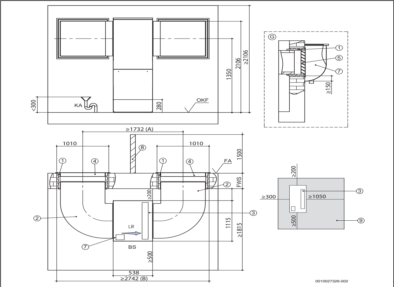
Bild 44 Kanalpläne Variante 3
