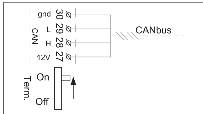
Bild 32 CAN-BUS-Terminierung
