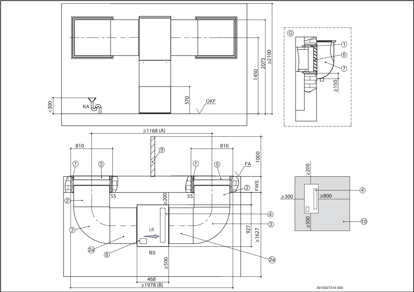
Bild 40 Kanalpläne Variante 2
