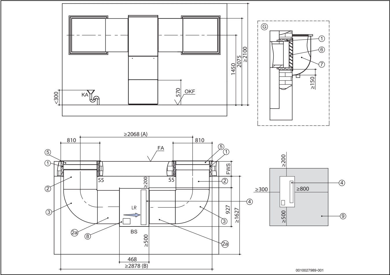
Bild 41 Kanalpläne Variante 3
