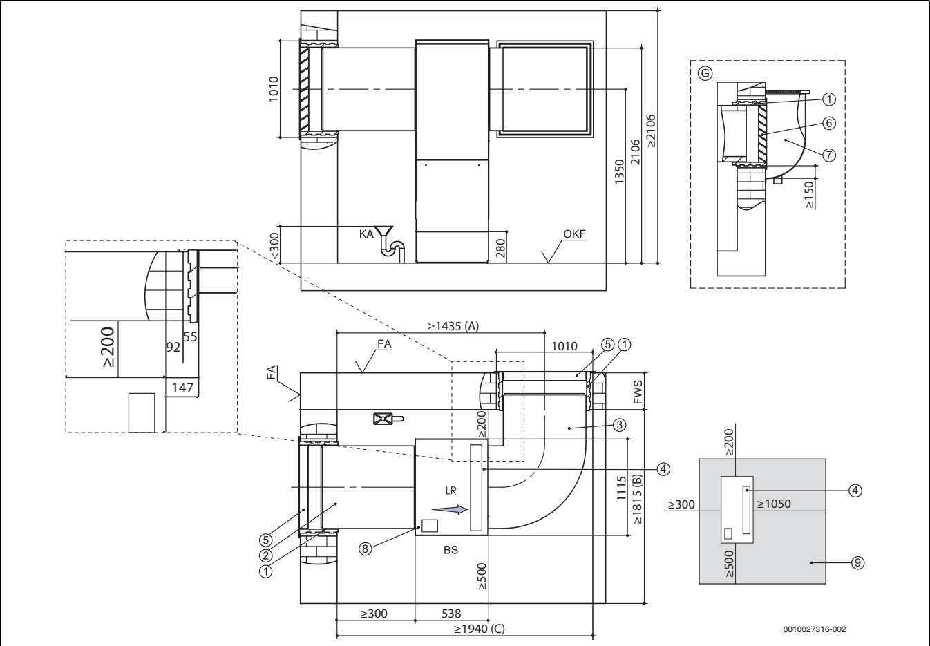
Bild 42 Kanalpläne Variante 1
